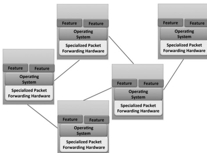
Рис. 1 -Традиційна мережева парадигма
