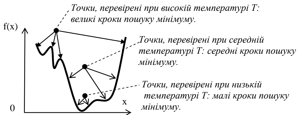
Рис. 11.5.9. Знаходження глобального мінімуму за методом «відпалу»
