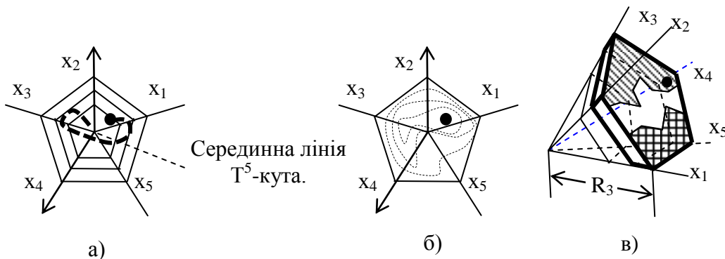
Рис. 2.3.16. Годограф (а), ізолінії (б) та визначені експертом граничні лінії станів об'єктів (в) на двовимірній мапі п'ятивимірного вхідного вектора R_3 (в) в одному T^5 -куті з його розділом сферами різних радіусів на три T^5_{g;r} -комірки при r=1, 2, 3
