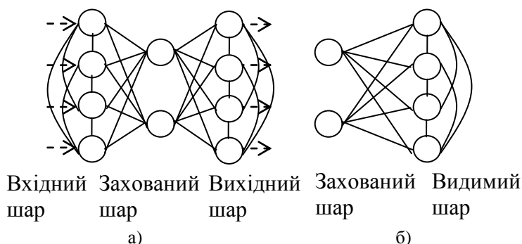
Рис. 11.5.8. Структура машини Больцмана: а) повнозв'язана; б) з обмеженням зв'язків
