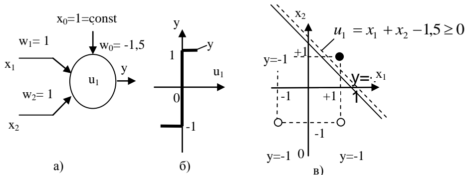
Рис. 8.2.1. Функція AND нейрону Adaline: а) схема; б) вихідна функція; в) геометричне пояснення
