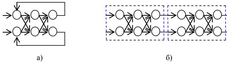
Рис. 11.7.1. Рекурсивна НМ зі зворотним поширенням сигналів
