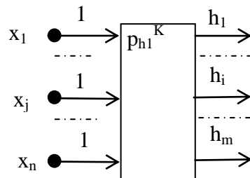
Рис. 11.5.10. Нейрон Байєса для віднесення об'єкта
