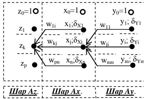
Рис. 9.5.2. Фрагмент схеми заміщення НМ (три шари багатошарової НМ) для розрахунку проходження похибок у зворотному напрямку від кінцевого шару до початкового вхідного шару на другому етапі
