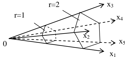
Рис. 2.3.3. Дві комірки 5-вимірного простору ( T_{g;r=1}^n та T_{g;r=2}^n )
