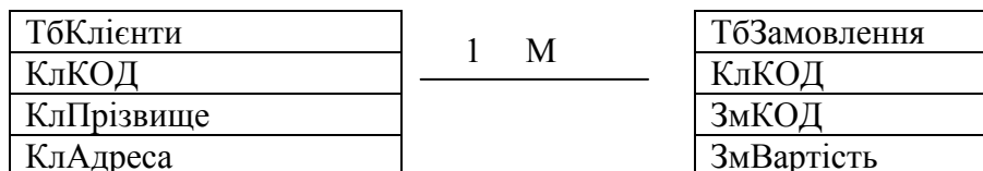
Рис. 4.12.4. Зв'язок «один-до-багатьох»
