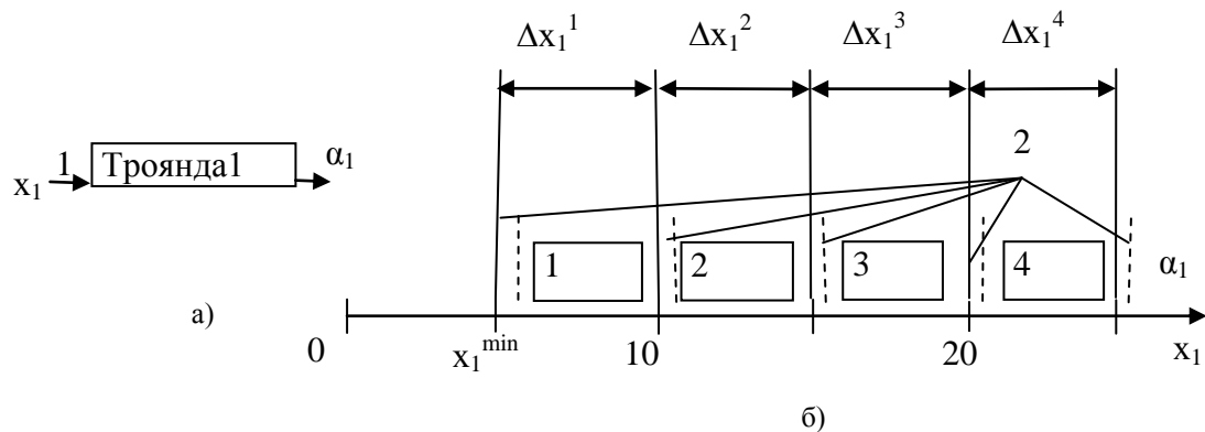
Рис. 10.1.5. Нейрон «Троянда1»
