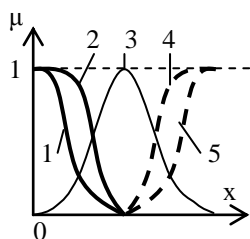
Рис. 4.7.3. Функції впевненості для термів:
