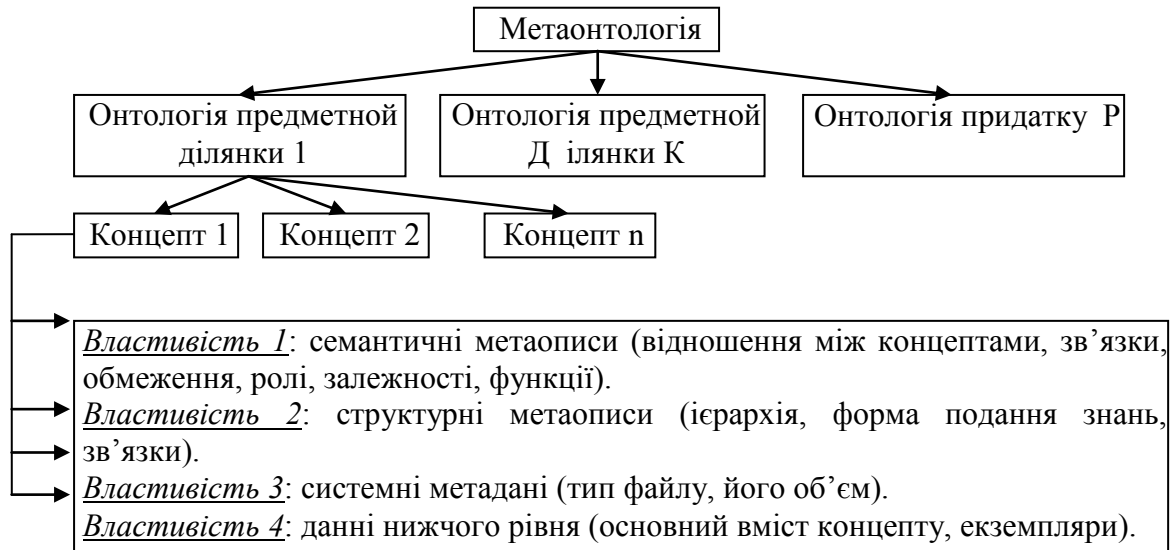
Рис. 13.2.2. Структура онтології
