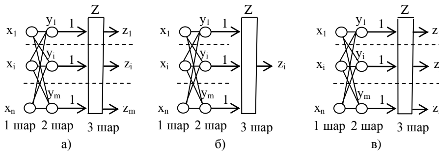
Рис. 11.2.8. Нейронні мережі:
