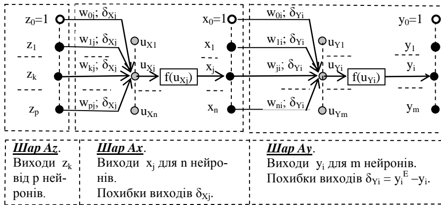
Рис. 9.5.1. Фрагмент схеми заміщення НМ (три шари багатошарової НМ) для розрахунку прямого потоку сигналів від початкового вхідного шару до кінцевого шару на першому етапі
