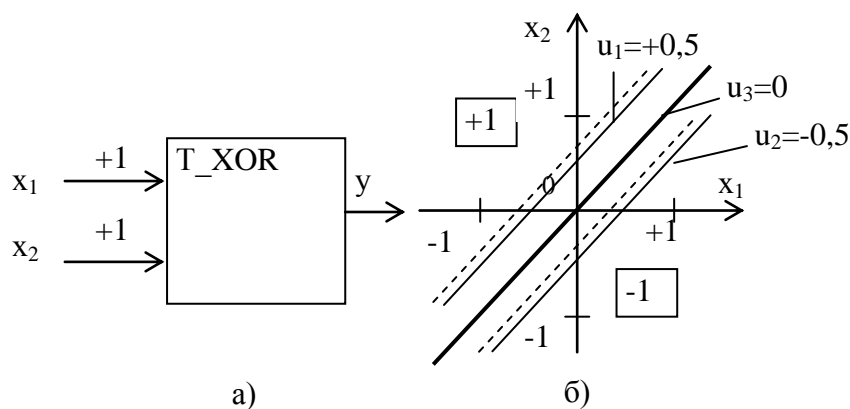
Рис. 10.1.9. Нейрон T_XOR
