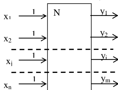
Рис. 10.6.1. Нейрон «Формула»
