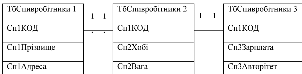
Рис. 4.12.3. Зв'язок 1:1 («один-до-одного»)
