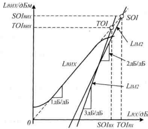
Рис. 9.9. Точки перетину другого (SOI) та третього (ТОІ) порядків Найвпливовішими вважаються компоненти із частотами f_{SOI} і f_{TOI} , які визначаються за формулами:
