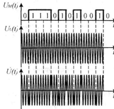
Рис. 7.17. Часова діаграма сигналу з BPSK
