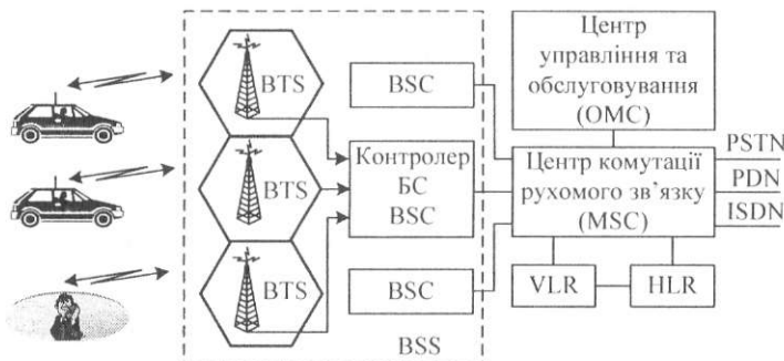
Рис. 8.22. Загальна структура мережі систем стільникового зв'язку GSM-900 і DCS-1800
