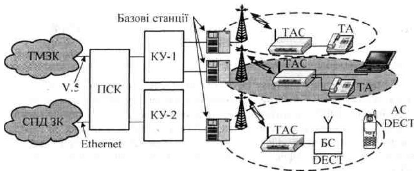
Структура системи радіодоступу
