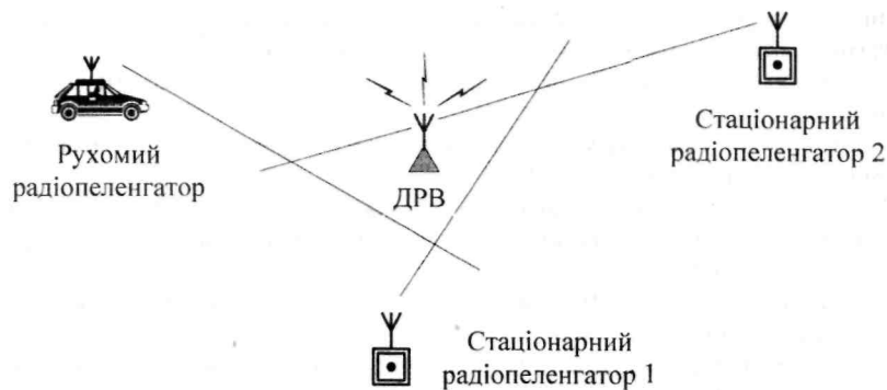
Рис. 5.3. Визначення місцезнаходження ДРВ триангуляційним методом
