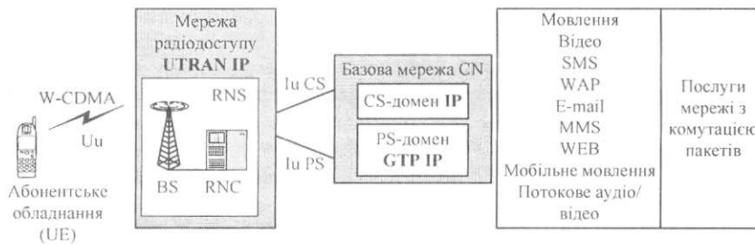
Рис. 8.30. Архітектура та послуги системи UMTS згідно з Release 6
