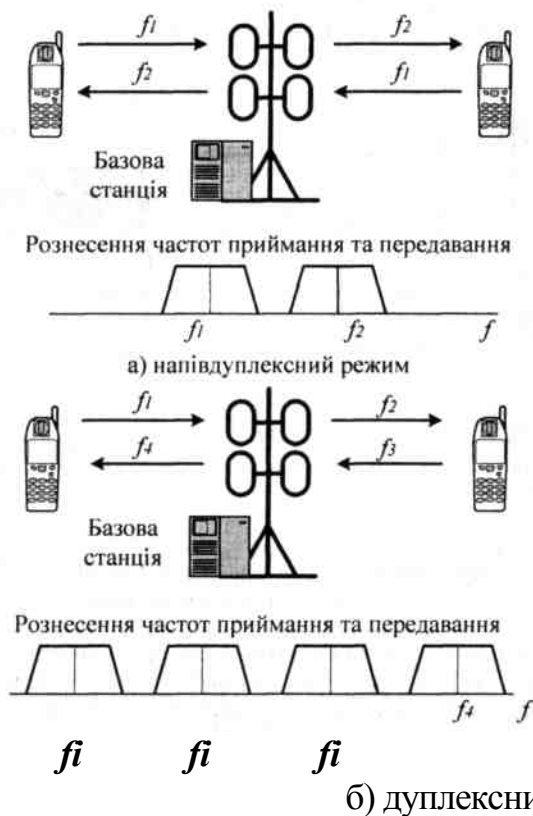
Рис. 8.63. Принцип рознесення частоту напівдуплексному та дуплексному режимах роботи
