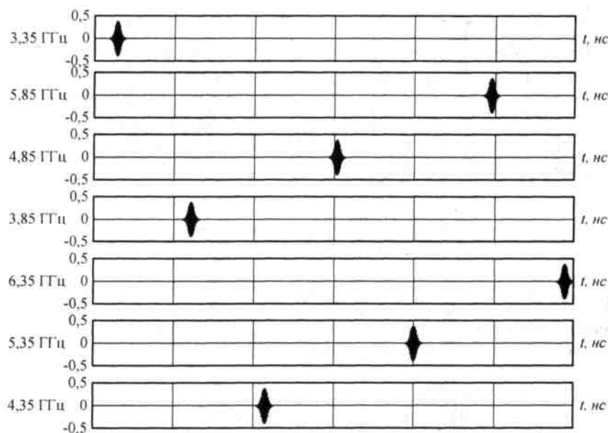
Рис. 8.95. Представлення послідовності імпульсів у частотній області
