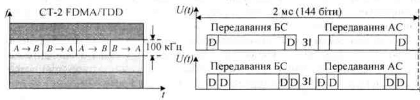
Рис. 8.55. Структура кадрів у стандарті СТ-2
