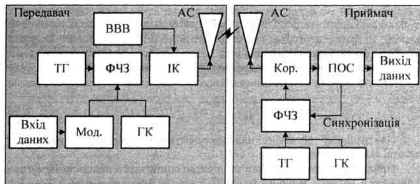
Рис. 8.90. Структурна схема системи Фулертон
