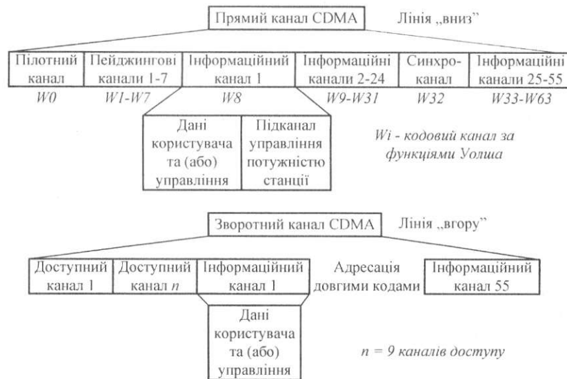
Рис. 8.36. Структура кадрів дуплексного радіоканалу в системі CDMA-800
