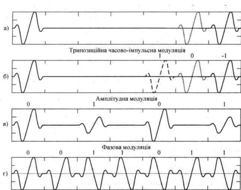
Рис. 8.89. Приклад часово-імпульсної, амплітудної та фазової модуляцій у засобах радіотехнології UWB
