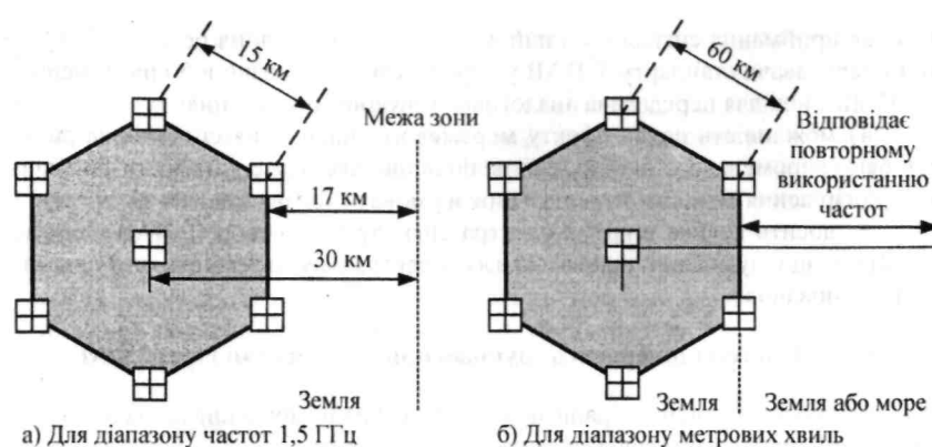
Рис. 8.10. Рекомендовані структури мереж T-DAB
