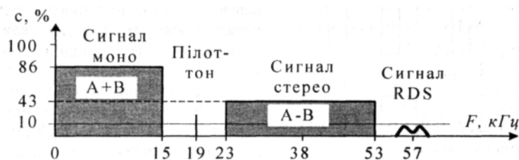
Рис. 8.67. Спектр сумарного сигналу (комплексного стереофонічного із сигналом RDS)
