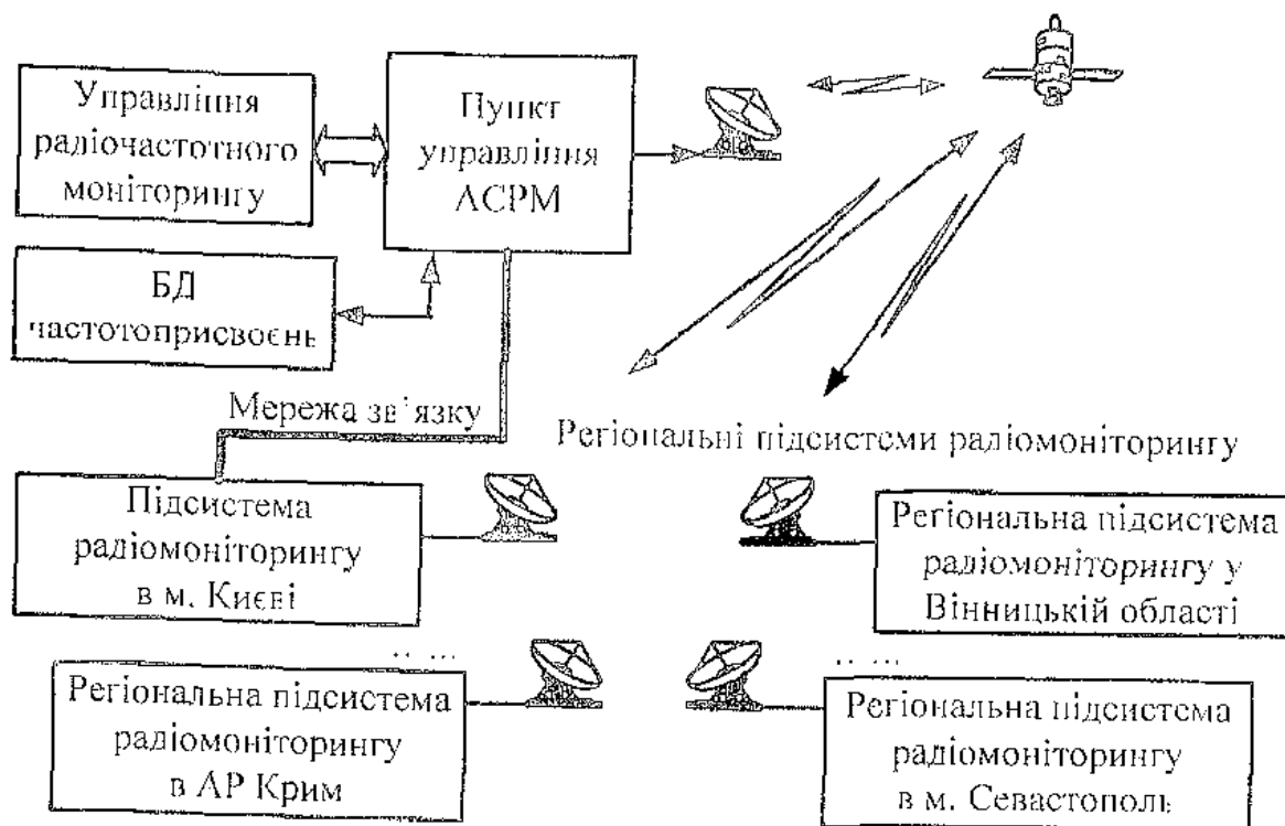
Рис. 10.9. Загальна структура АСРМ УДЦР
