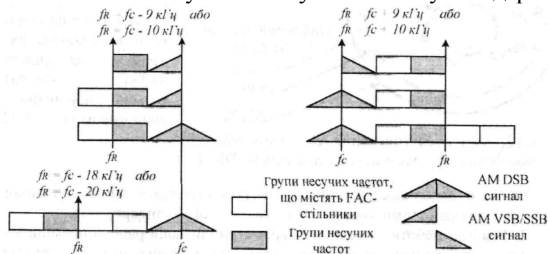
Рис. 8.13. Розташування несучих частот у стандарті DRM
