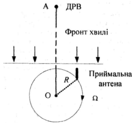
Рис. 5.16. Процес зміни фази коливань у радіопеленгаторі з використанням ефекту Доплера
