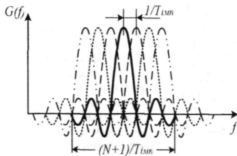
Рис. 7.27. Принцип модуляції OFDM
