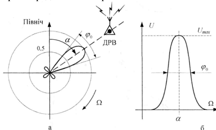
Рис. 5.9. Принцип пеленгування за максимальним значенням сигналу
