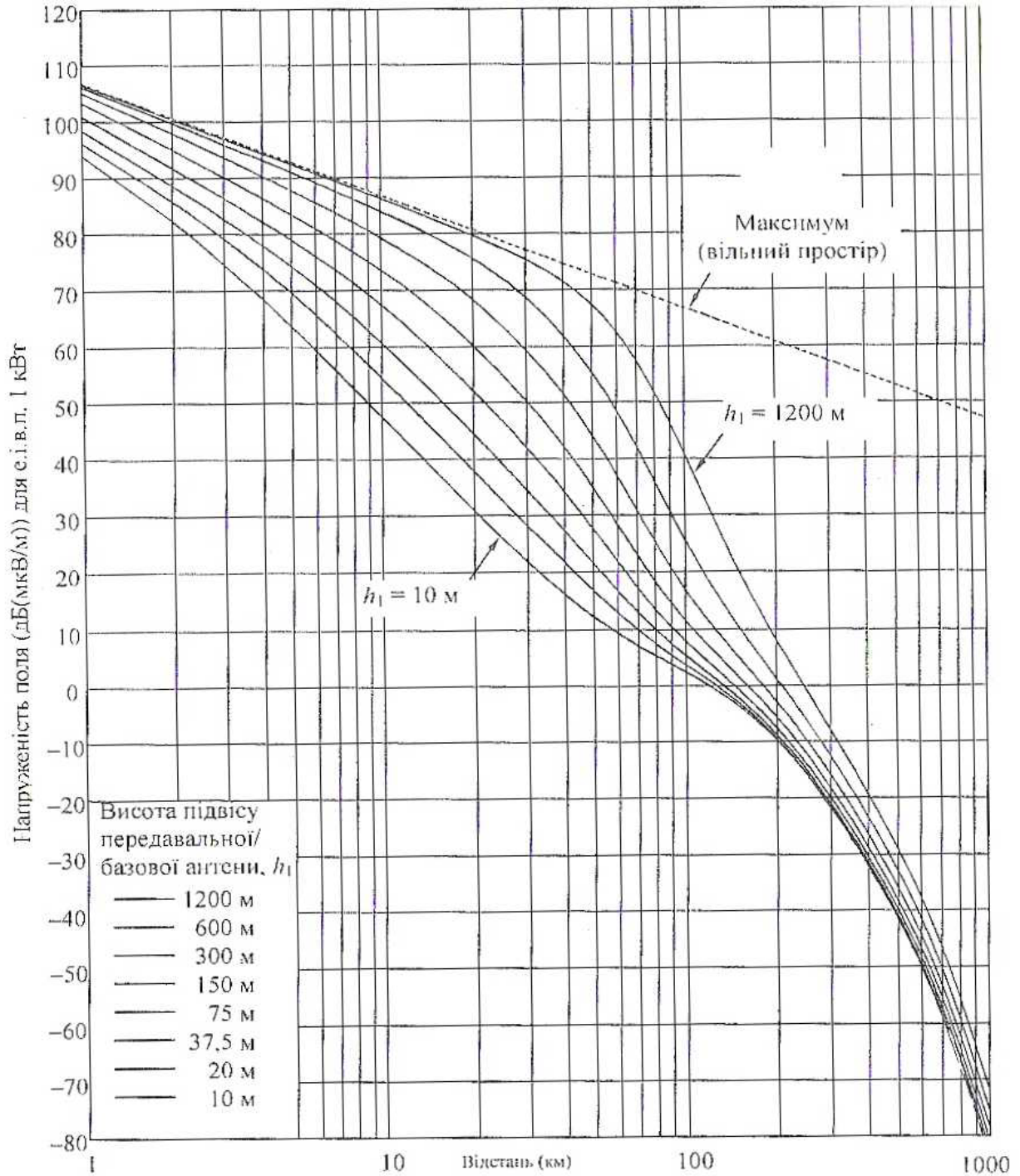
Рис. 10.12. Крива поширення для частоти 2000 МГц (сухопутна траса, 50 % часу)
