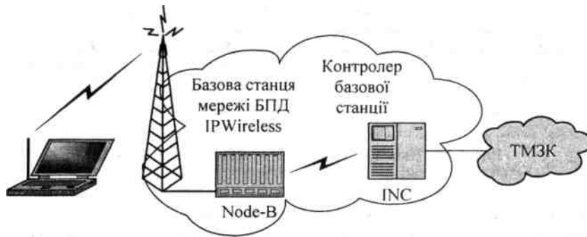
Рис. 8.87. Загальна структура мережі IPWireless
