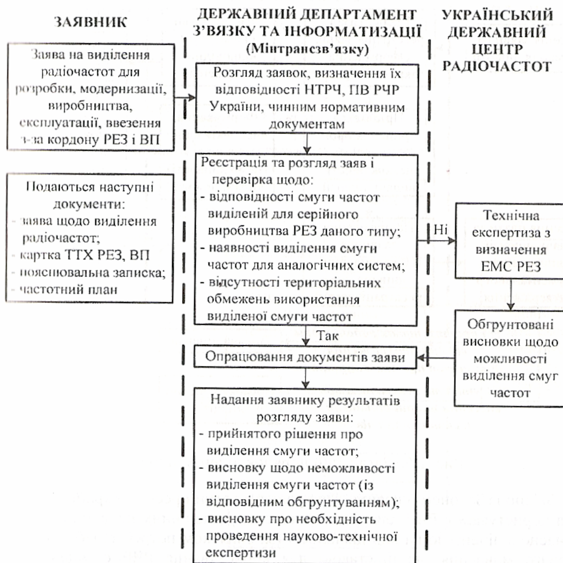
Рис. 2.4. Порядок виділення смуг радіочастот
