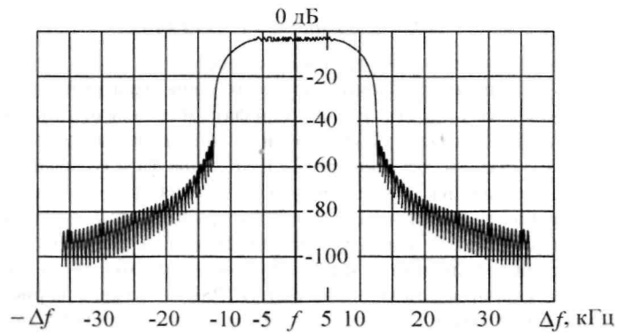
Рис. 7.20. Теоретичний спектр сигналу DQPSK
