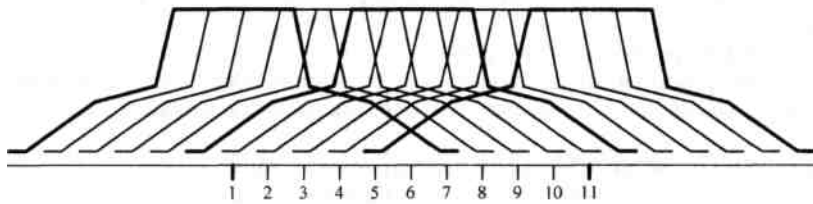
Рис. 8.74. Загальний принцип розподілу каналів за стандартом IEEE 802.11b
