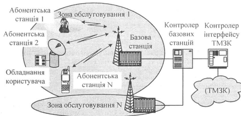
Рис. 8.32. Структура системи радіодоступу в мережах зв'язку систем CDMA-800 і CDMA-450
