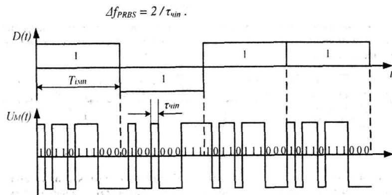
Рис. 7.6. Модуляція цифрового потоку розширювальним кодом
