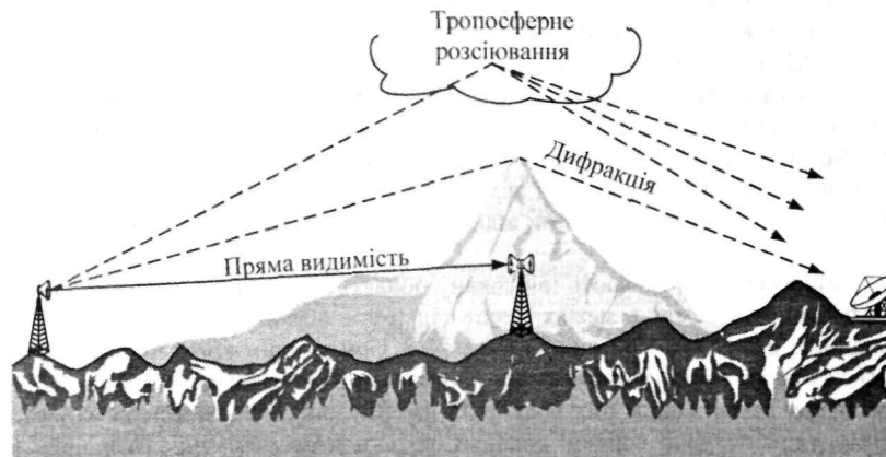
Рис. 6.2. Короткочасні механізми поширення радіохвиль
