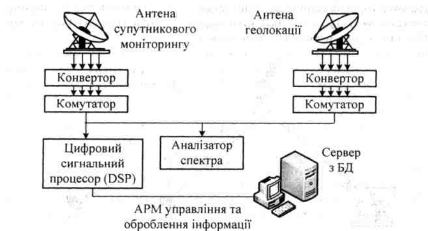
Рис. 8.54. Структурна схема станції геолокації земних станцій супутникового зв'язку
