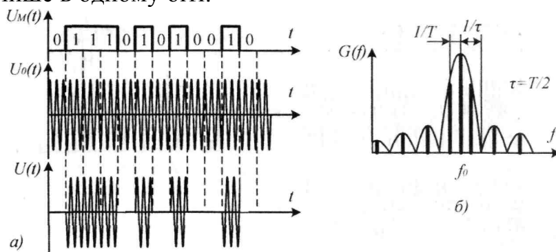
Рис. 7.11. Часовий графік і спектр АМн сигналу. Сигнальне сузір'я АМн сигналу зображене на рис. 7.12.
