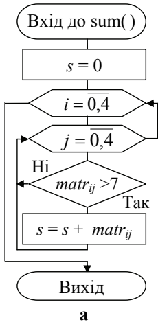
Блок-схеми функцій: а – sum(); б – zamina()
