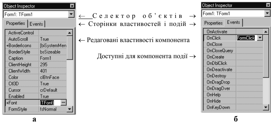
Рис. 2.5. Вікна інспектора об'єктів:
