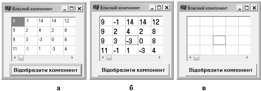
Рис. 14.4. Результати роботи з компонентом SGt:
