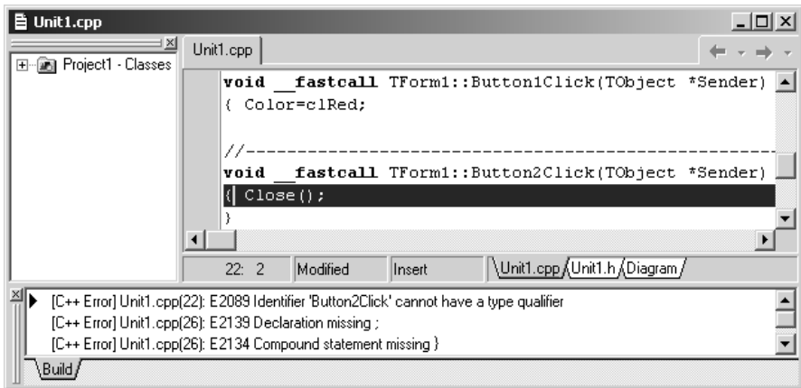
Рис. 15.6. Помилка E2089: пропущено закриту дужку у попередній функції
