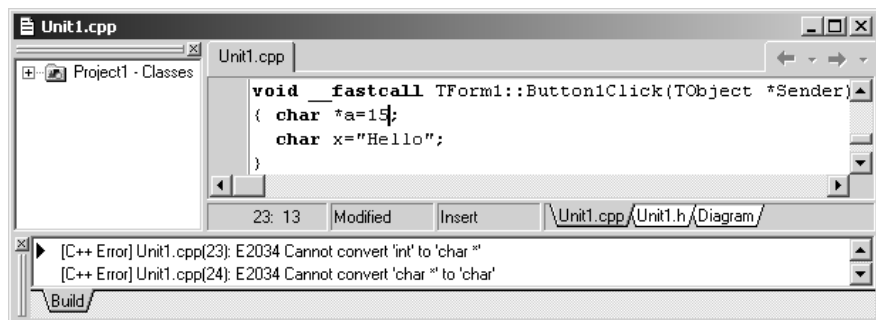
Рис. 15.17. Помилка E2034: суперечка типів
