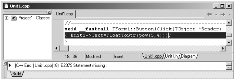
Рис. 15.2. Помилка E2379: зайва дужка у математичному виразі
