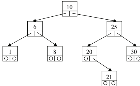
Рис. 13.1. Приклад зображення бінарного дерева
