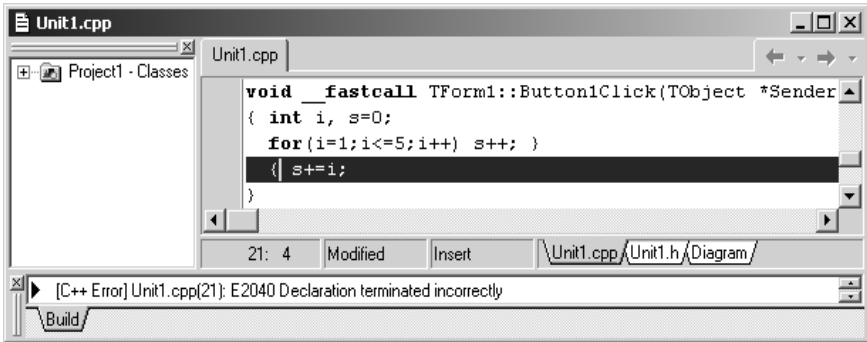
Рис. 15.18. Помилка E2040: фігурна дужка закрита завчасно
