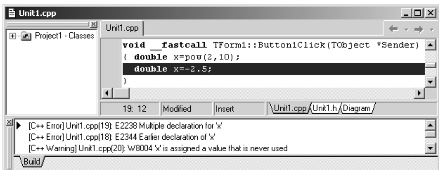
Рис. 15.9. Помилка E2238: змінну x оголошено двічі
