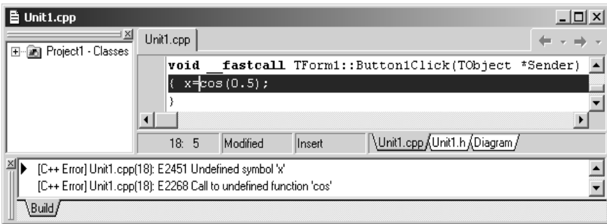
Рис. 15.7. Помилка E2451: не оголошено змінну x
