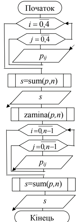
Блок-схема основної програми (кнопка “Розв’язок”)
