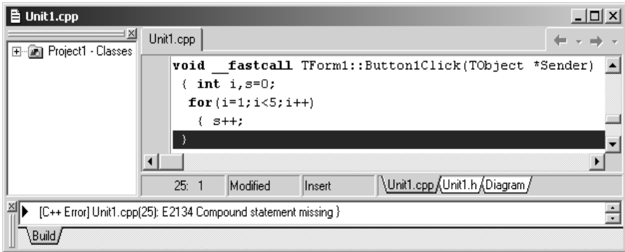
Рис. 15.10. Помилка E2134: пропущено закриту фігурну дужку
