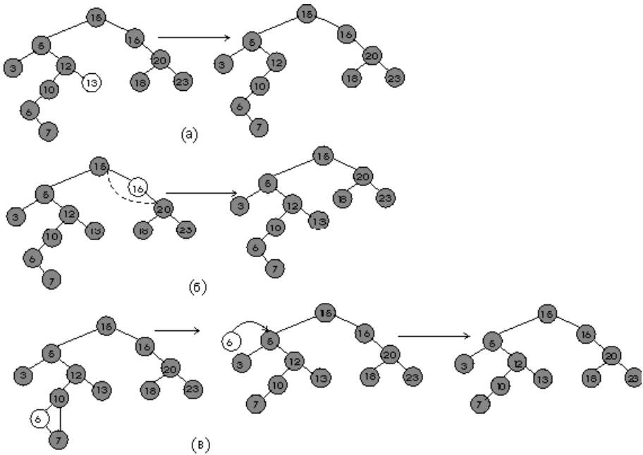
Рис. 13.2. Різні випадки вилучення вузлів дерева:
