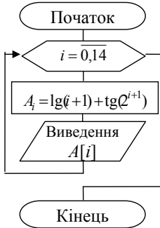
Блок-схема для кнопки “Обчислення вектора”
