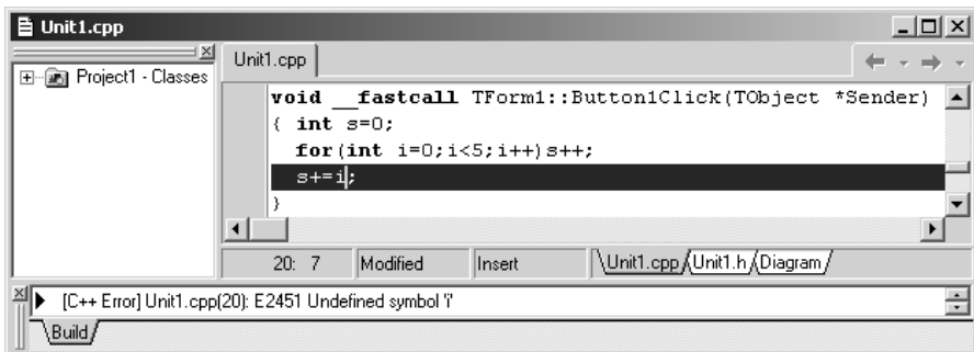
Рис. 15.8. Помилка E2451: змінну s оголошено в іншій області видимості
