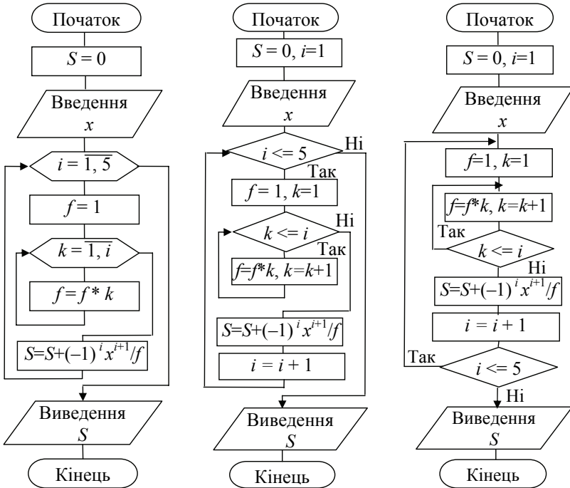
а б в Схеми алгоритмів програм з різними операторами циклу: а – for; б – while; в – do-while
