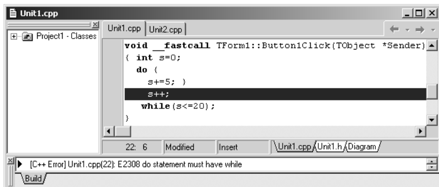
Рис. 15.20. Помилка E2308: завчасно закрито фігурну дужку
