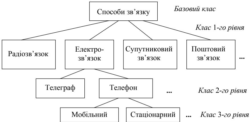
Рис. 14.1. Ієрархія класів “Способи зв’язку”
