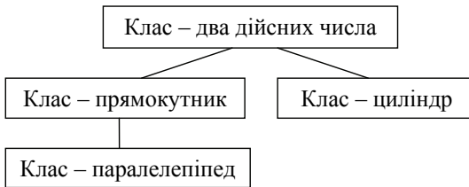
Рис. 14.2. Ієрархія класів для прикладу 14.5
