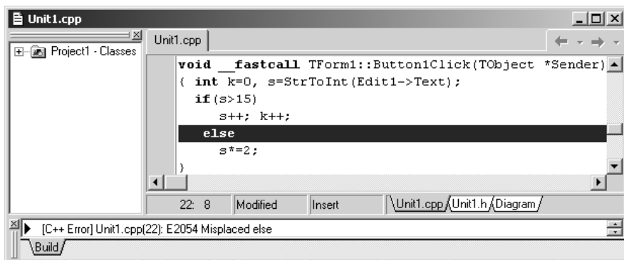
Рис. 15.16. Помилка E2054: неможливо встановити, до якого if належить else, через те, що пропущено фігурні дужки
