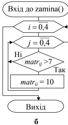
Блок-схеми функцій: а – sum(); б – zamina()
