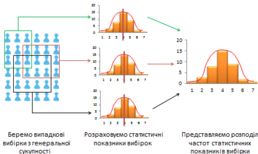
Рис. 8.3. Розподіл вибірок
