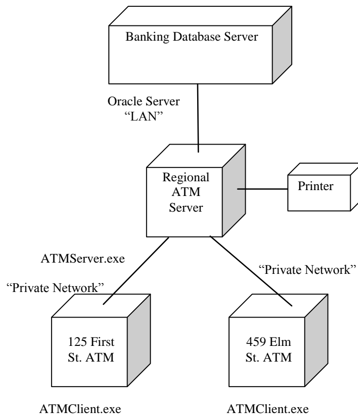
Рисунок 4.19. Приклад діаграми розміщення
