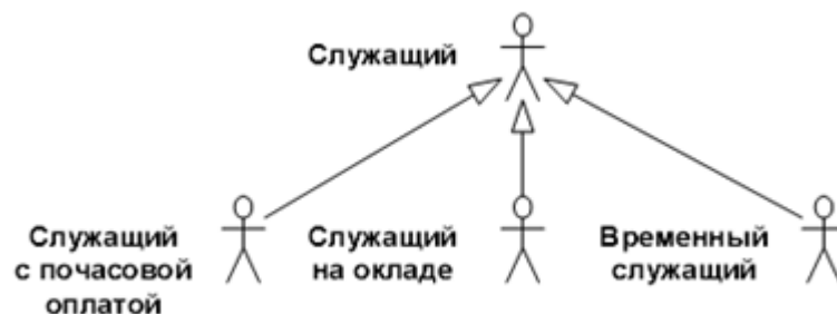
Рисунок 4.6. Приклад зв'язку узагальнення
