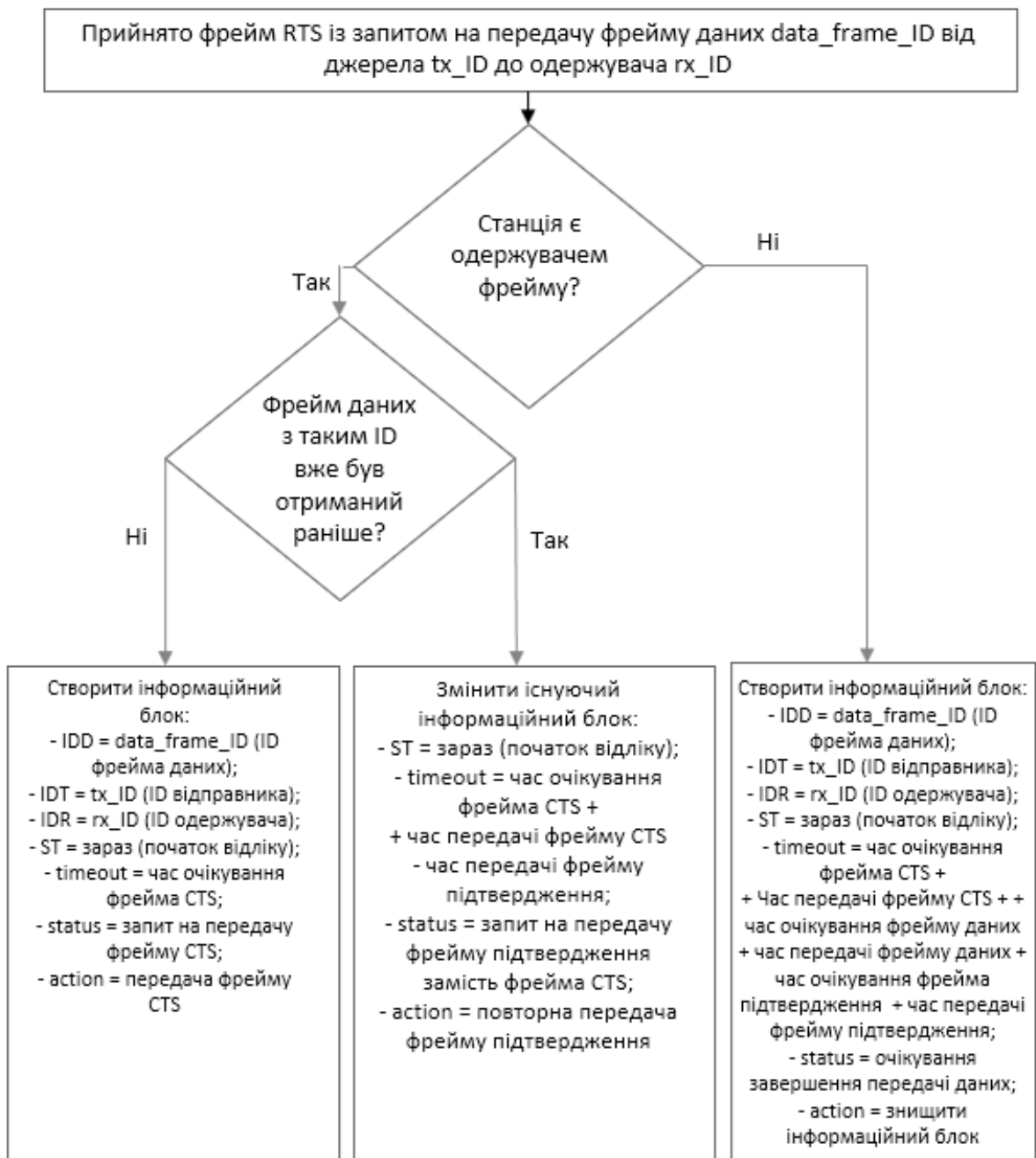
Рис. 2.18. Отримання фрейму RTS
