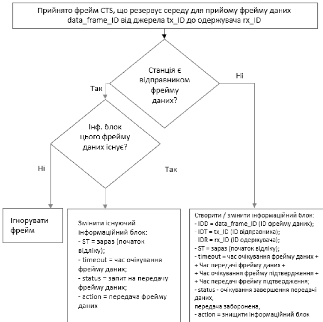
Рис. 2.19. Отримання фрейму CTS
