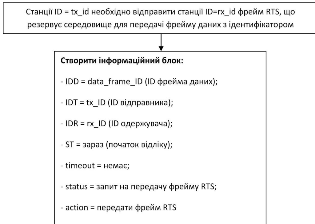
Рис. 2.14. Запит на відправку фрейму RTS
