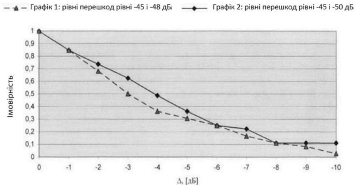
Рис. 2.3. Результати розрахунків сумарного рівня перешкод
