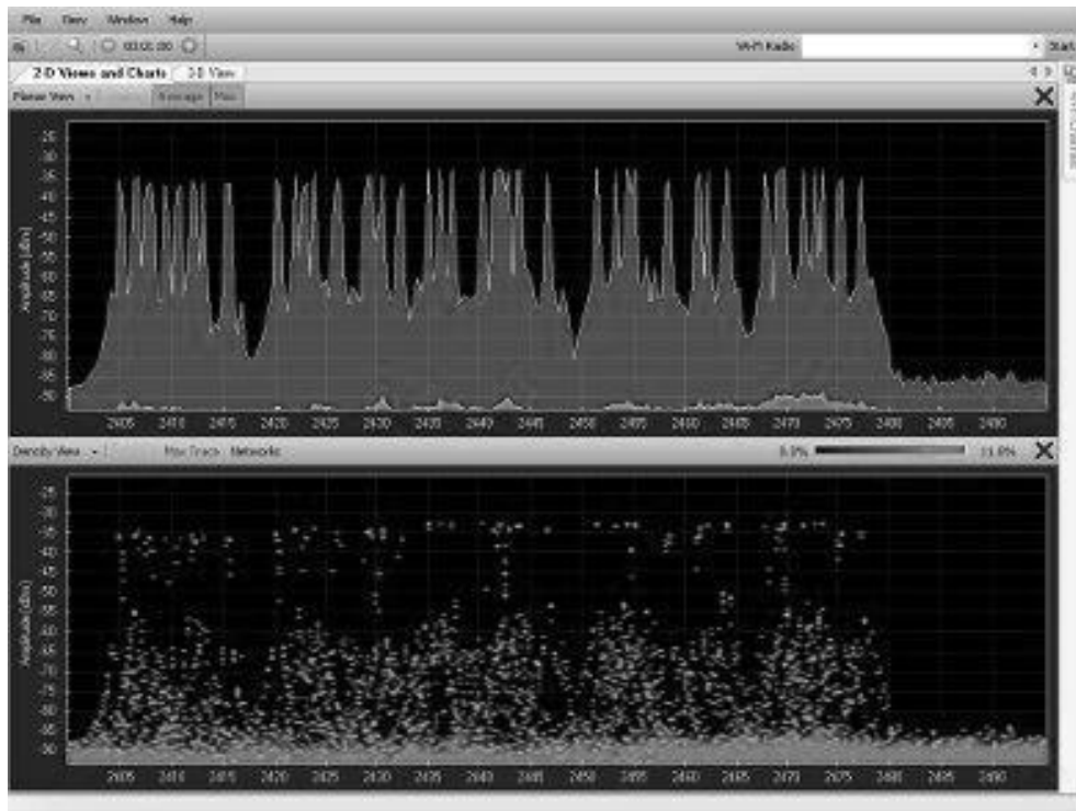
Рис. 3.3. Спектр FHSS-сигнала
