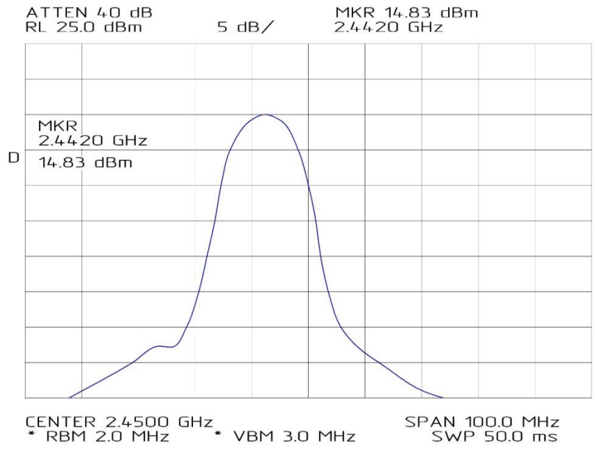
Рис. 2.8. D-Link DWL810
