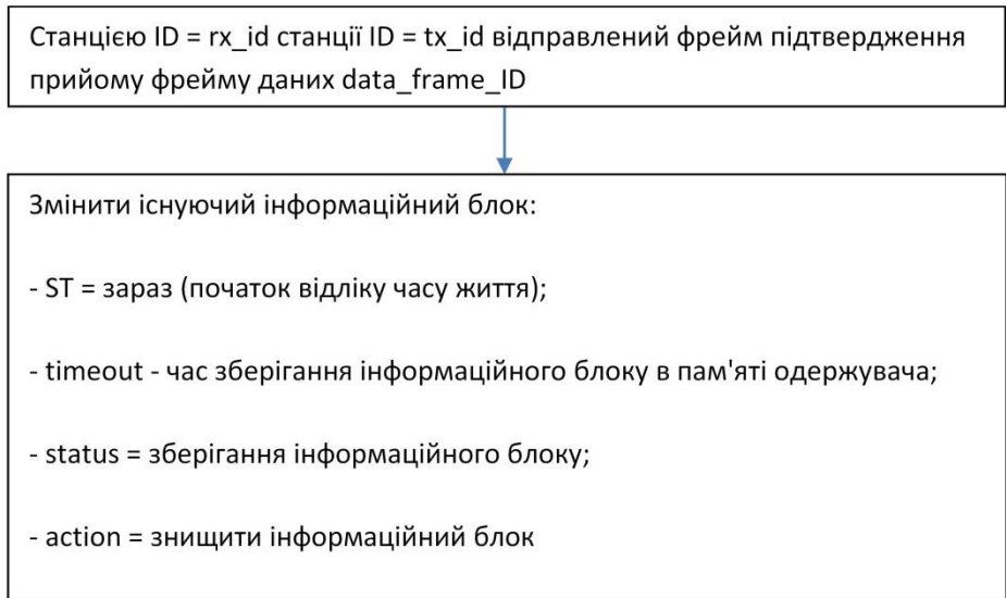
Рис. 2.21. Відправка фрейму підтвердження
