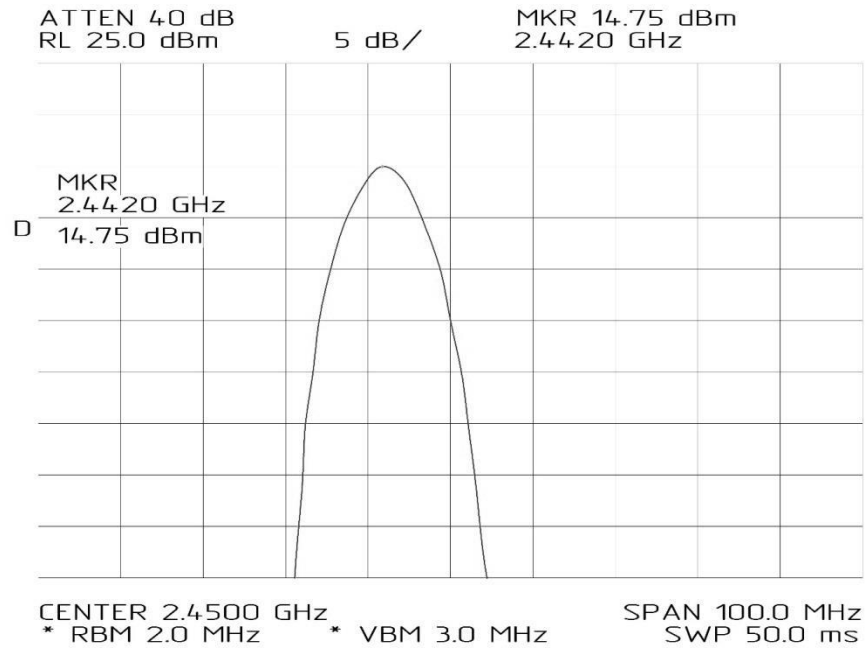
Рис. 2.12. Orinoco
