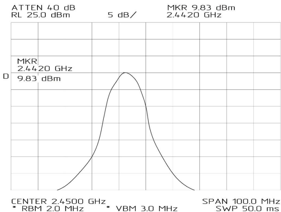
Рис. 2.7. D-Link DWL650
