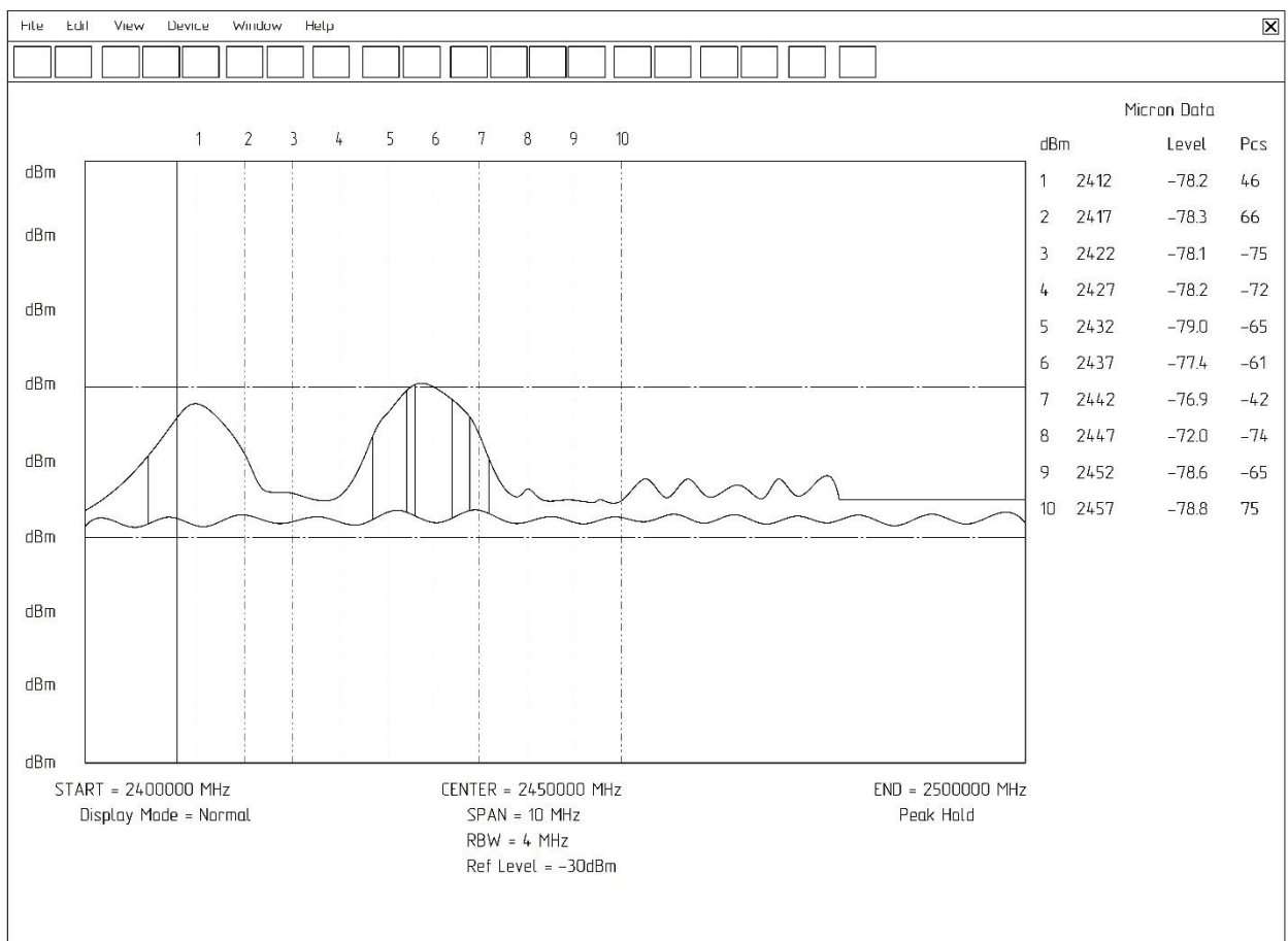
Рис. 3.2. Спектр DSSS-сигналу
