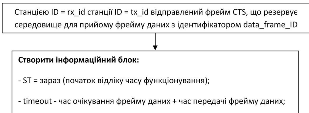
Рис. 2.17. Відправка фрейму CTS
