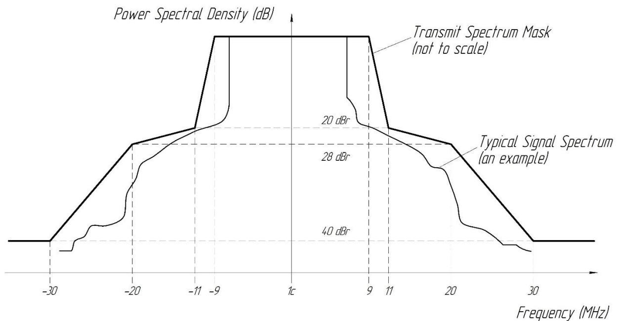
Рис. 2.5. Спектральна маска
