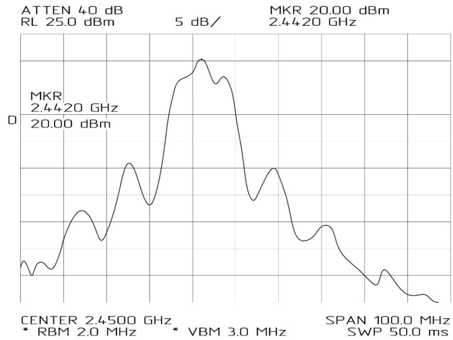
Рис. 2.11. BreezeCom DS.11
