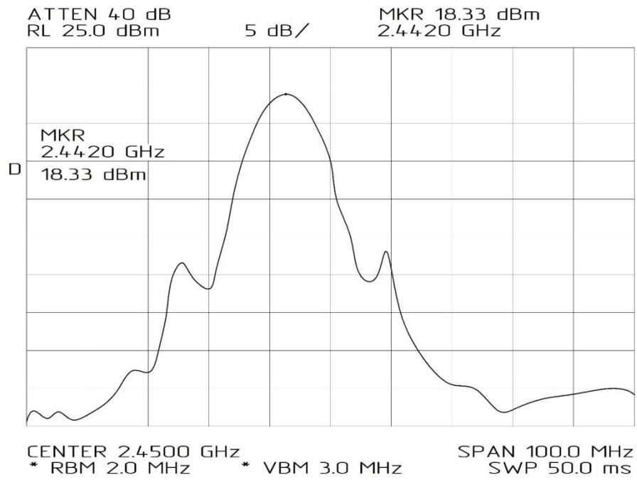
Рис. 2.10. AirBridge
