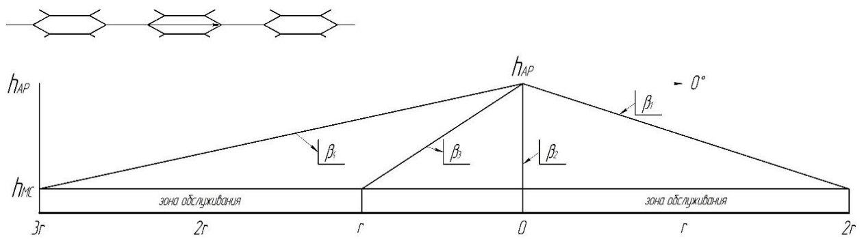
Рис. 3.7. Вимоги до вертикальної ДС антени АР
