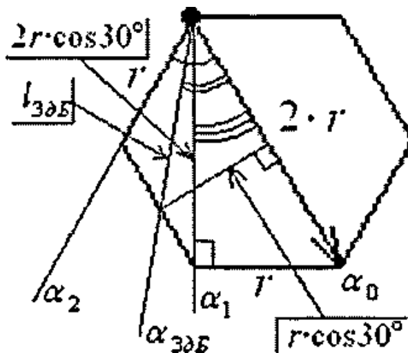
Рис. 3.6. Розташування антени AP і критичних МС
