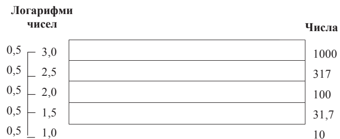
Рис. 12.9. Логарифмічна шкала
