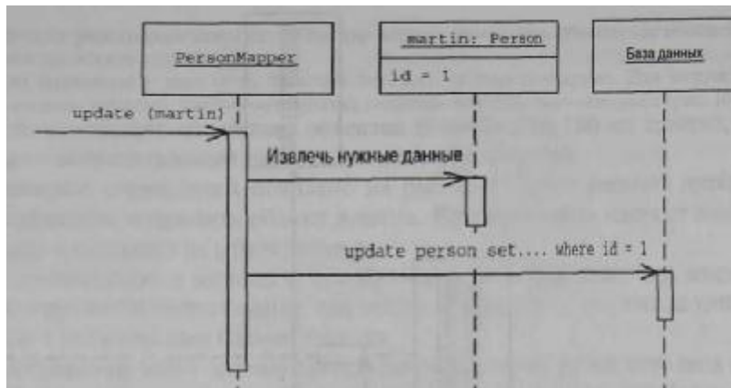
Рис. 10.4. Обновление данных
