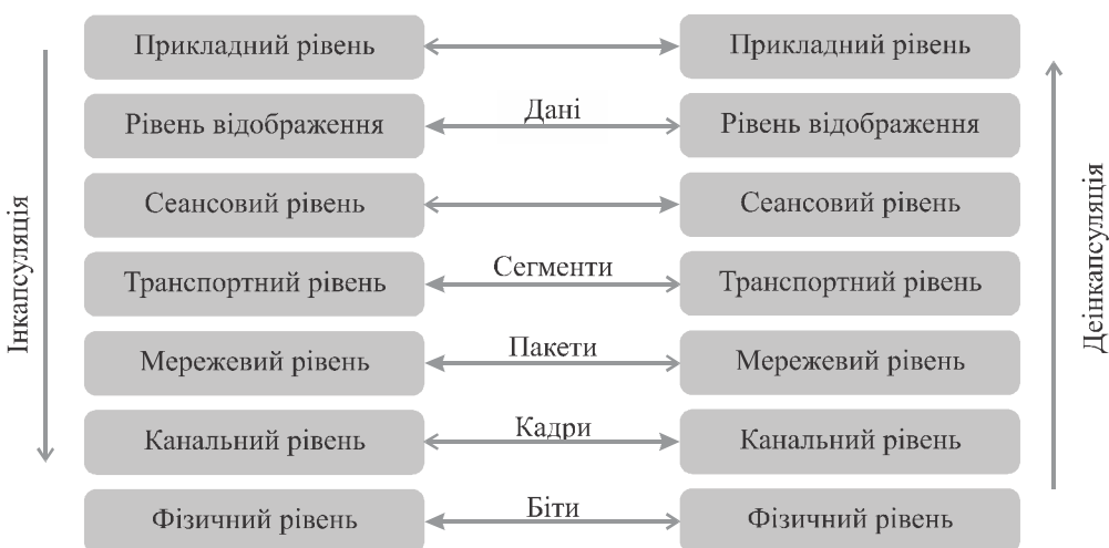
Рис. 1.4. Інкапсуляція даних
