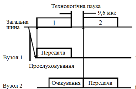
Рисунок 4.25. – Метод випадкового доступу CSMA/CD
