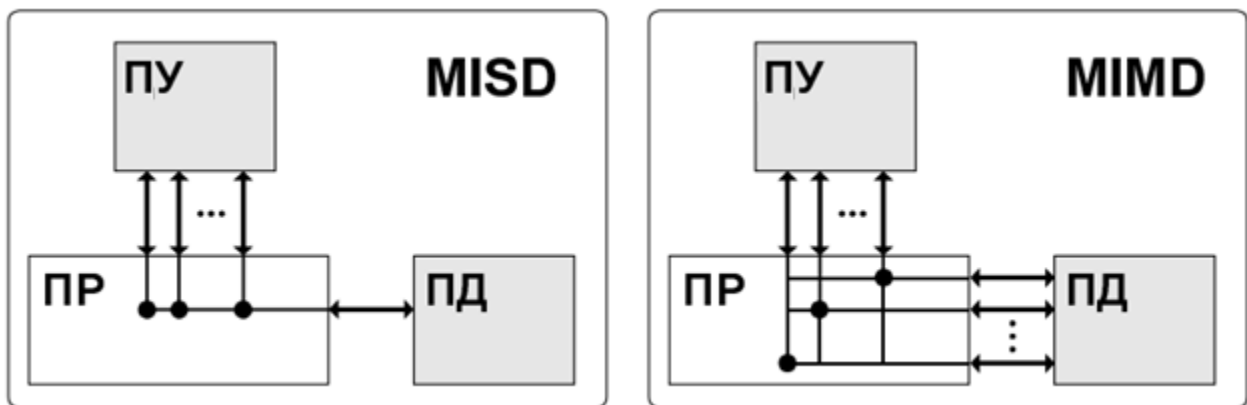
Рисунок 3.2. – Класи MISD і MIMD класу класифікації М. Флінна
