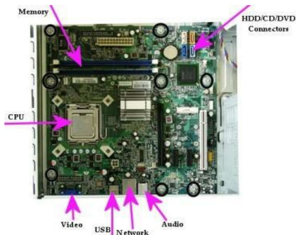
Рис. 2.8. Материнська плата
