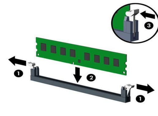
Рис. 2.12. Кроки встановлення модуля пам'яті
