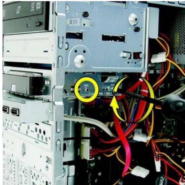
Рис. 3.8. Прикріплення ґвинтів
