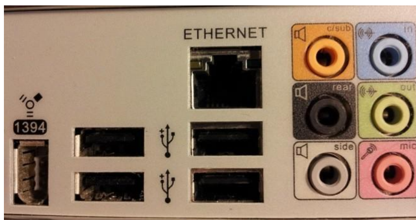
Рис. 2.14. Інтерфейси I/O
