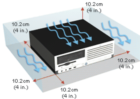
Рис. 2.6. Особливості вентиляції
