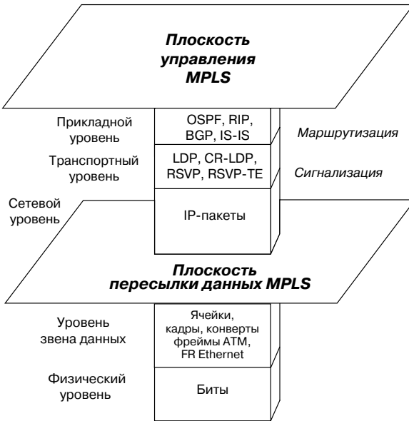
Рис. 1.1. Плоскости MPLS
