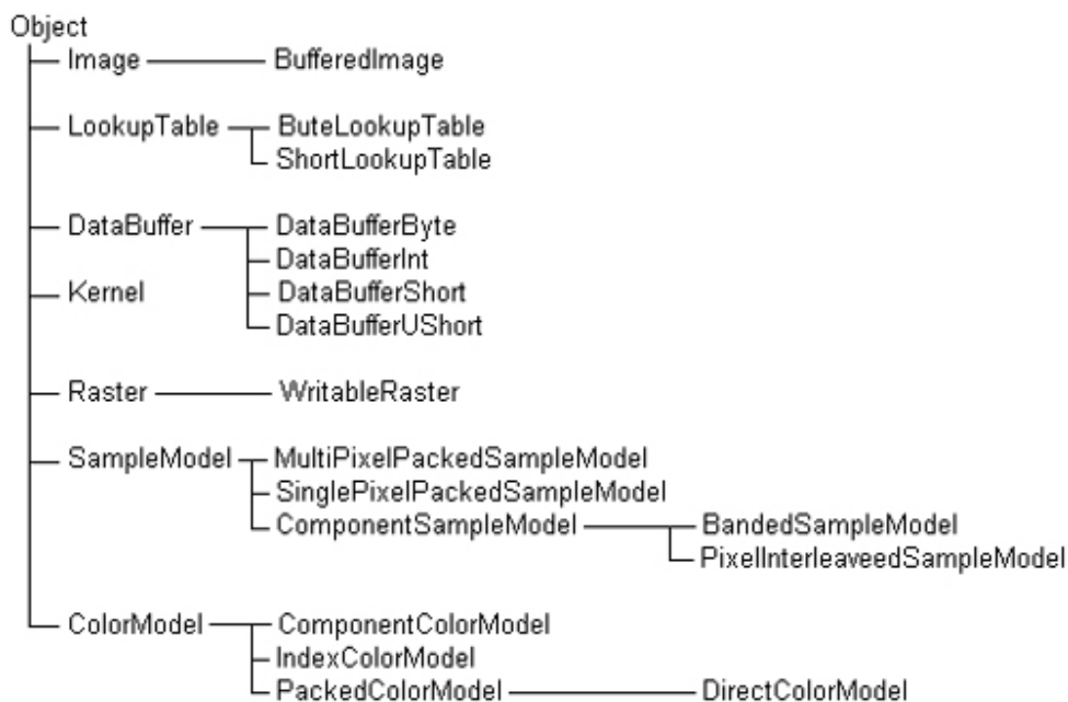
Рис. 15.5. Класи, реалізуючі модель прямого доступу
