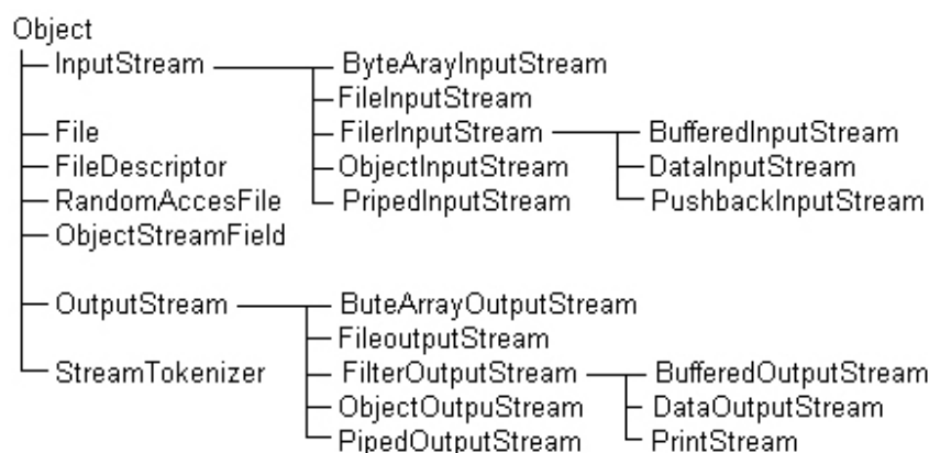
Рис. 18.2. Класи байтових потоків
