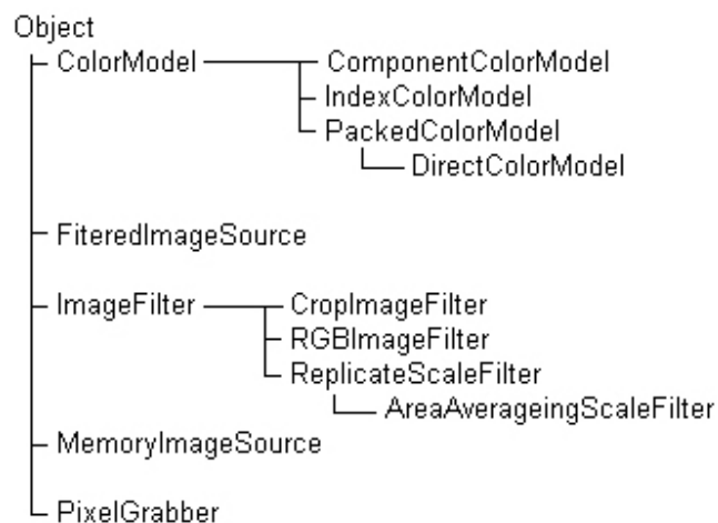
Рис. 15.2. Класи, реалізуючі модель "постачальник-споживач"
