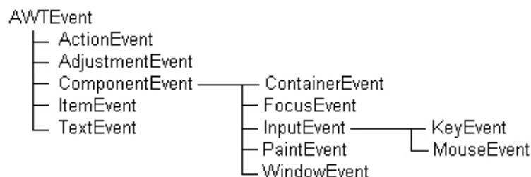
Рис. 12.1. Ієрархія класів, описуючих події AWT
