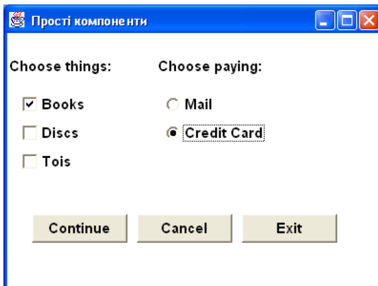
Рис. 10.1. Прості компоненти
