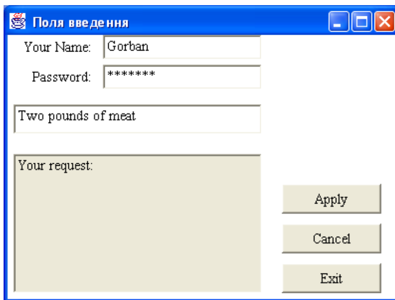
Рис. 10.3. Поля введення
