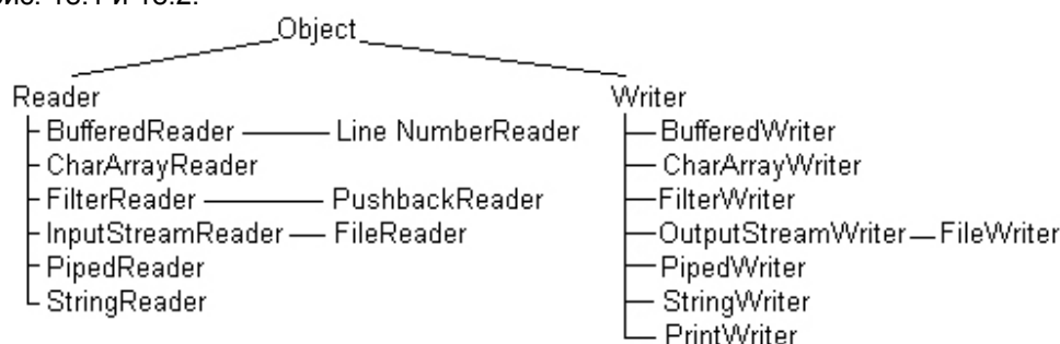
Рис. 18.1. Ієрархія символних потоків
