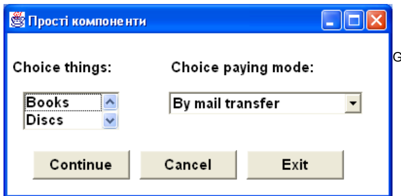
Рис. 10.2. Використання списків
