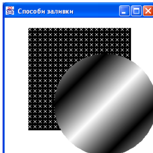
Рис. 9.5. Способи заливки
