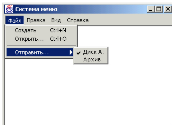
Рис. 13.1. Система меню
