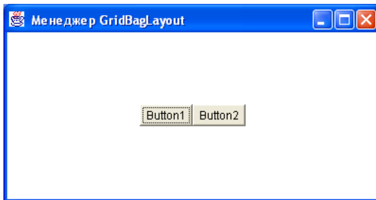
Рис. 11.6. Менеджер GridBagLayout
