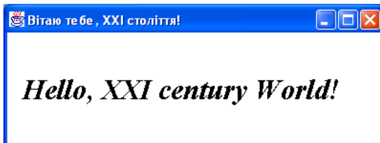
Рис. 8.1. Вікно програми-привітання
