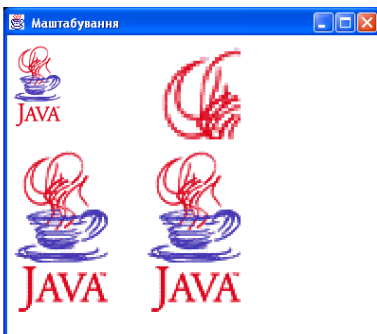
Рис. 15.3. Маштабування зображення
