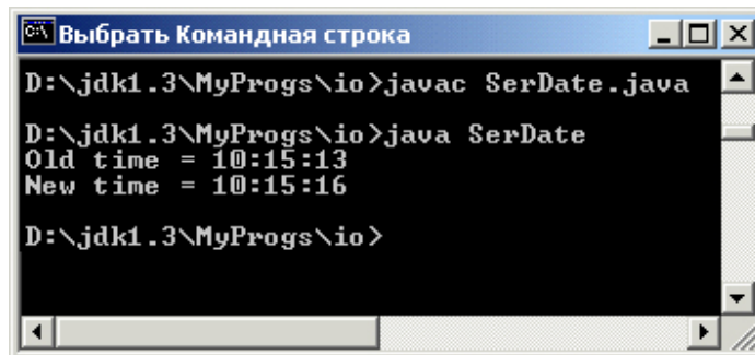
Рис.18.7. Серіалізація об'єкта
