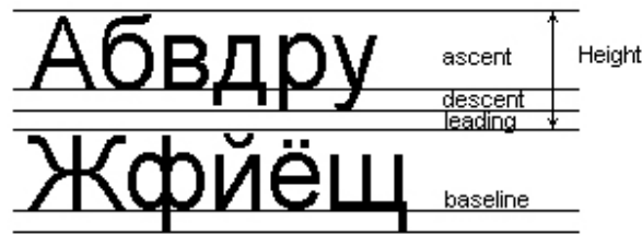
Рис. 9.1. Елементи шрифту
