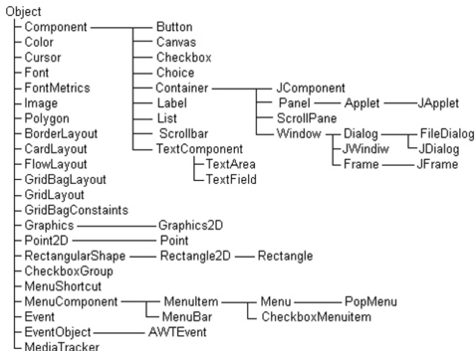
Рис. 8.2. Ієрархія основних класів AWT
