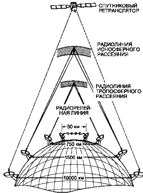
Рисунок 5.1 – Система супутикового зв'язку
