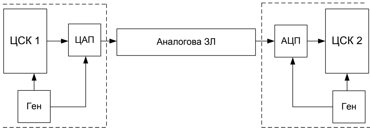
Рисунок 3.6 - 2 – й етап – 2 варіант – Цифрові системи комутації і аналогові системи передавання
