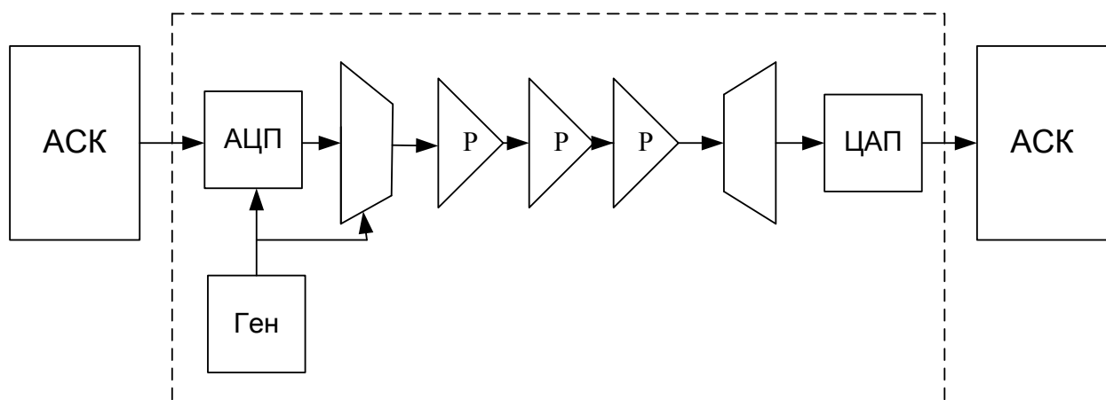
Рисунок 3.5 - 2 – й етап – 1 варіант – аналогові системи комутації і цифрові системи передавання.
