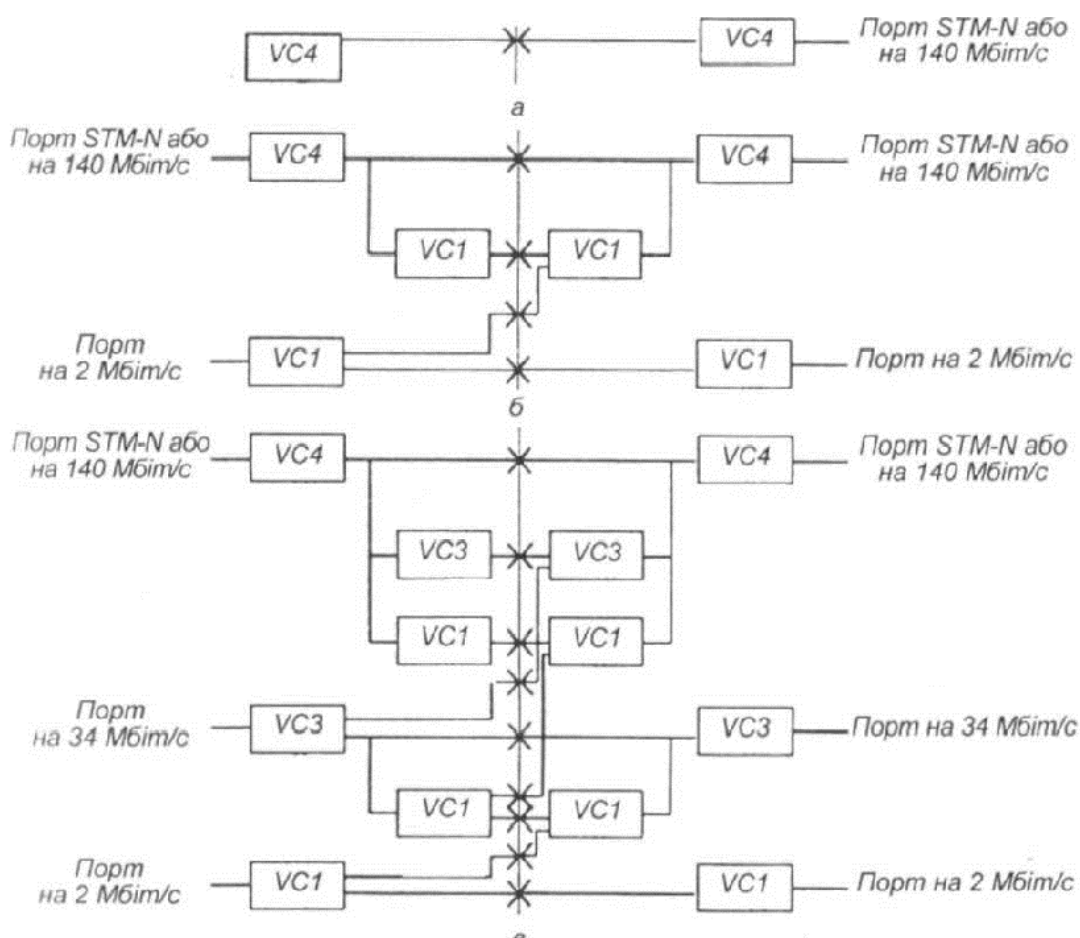
Рисунок 4.8 – Перемикання в апаратурі оперативного перемикавання 4/4 (а), 4/1 (б) та 4/3/1 (в)
