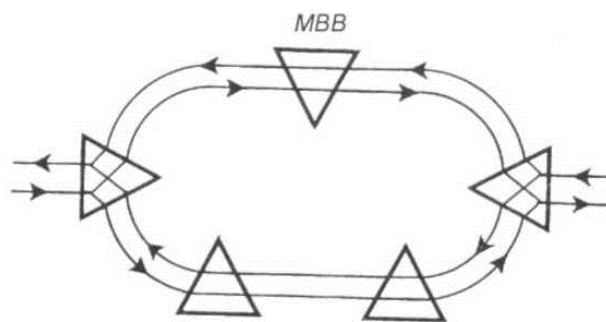
Рисунок 4.11 – Схема проходження сигналів за двома напрямками передавання інформації для одного з'єднання в односпрямованому кільці
