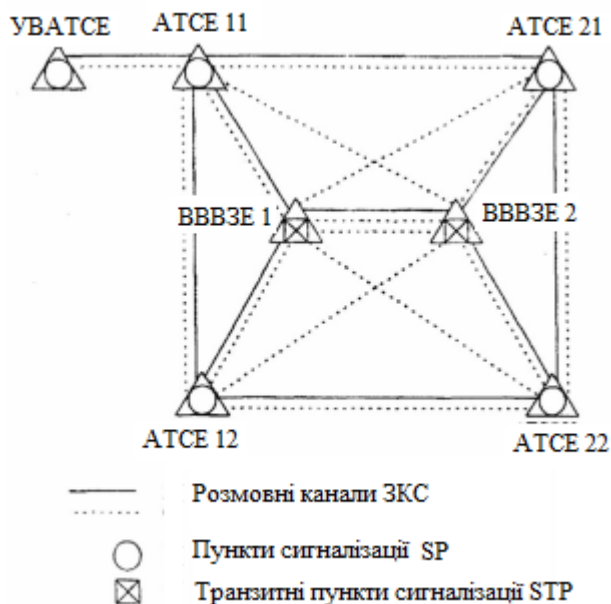
Рисунок 8.2 – Приклад ЗКС №7 на МТМ з вузлоутворенням
