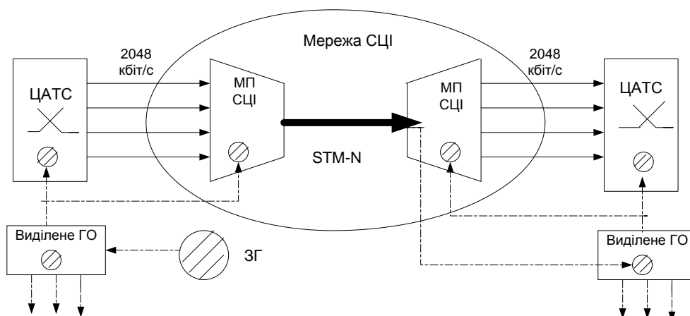
Рисунок 3.9 - Синхронізація двох цифрових вузлів комутації по лінії передавання СЦІ.
