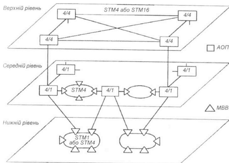
Рисунок 4.10 - Трирівнева архітектура мережі синхронної цифрової ієрархії
