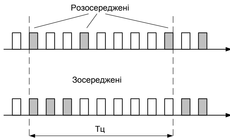
Рисунок 1.6 – Приклад багатосимвольної розосередженої та зосередженої синхрогруп
