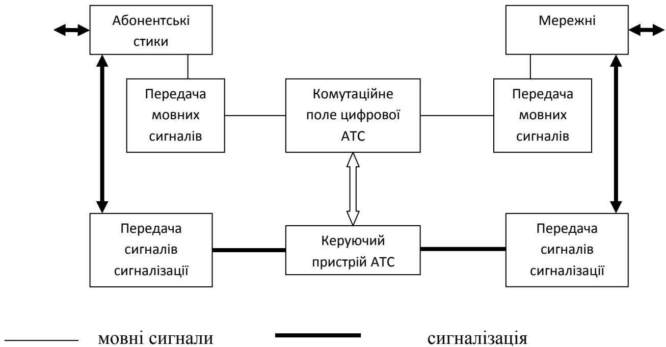
Рисунок 9.1 - Проходження мовних сигналів і сигналів сигналізації в цифровій АТС
