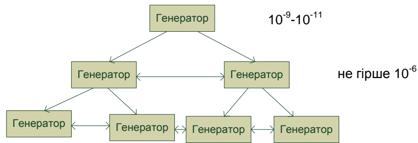
Рисунок 2.1 - Багаторівнева ієрархічна структура взаємодії тактових генераторів мережі
