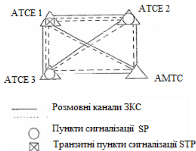
Рисунок 8.1 – Приклад ЗКС №7 на МТМ без вузлоутворення
