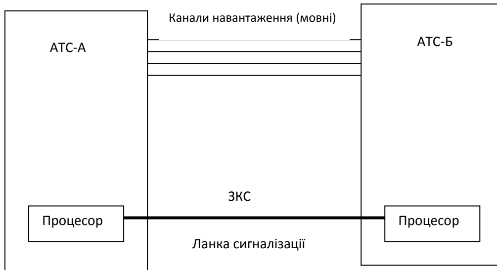
Рисунок 7.1 – Використання ЗКС №7
