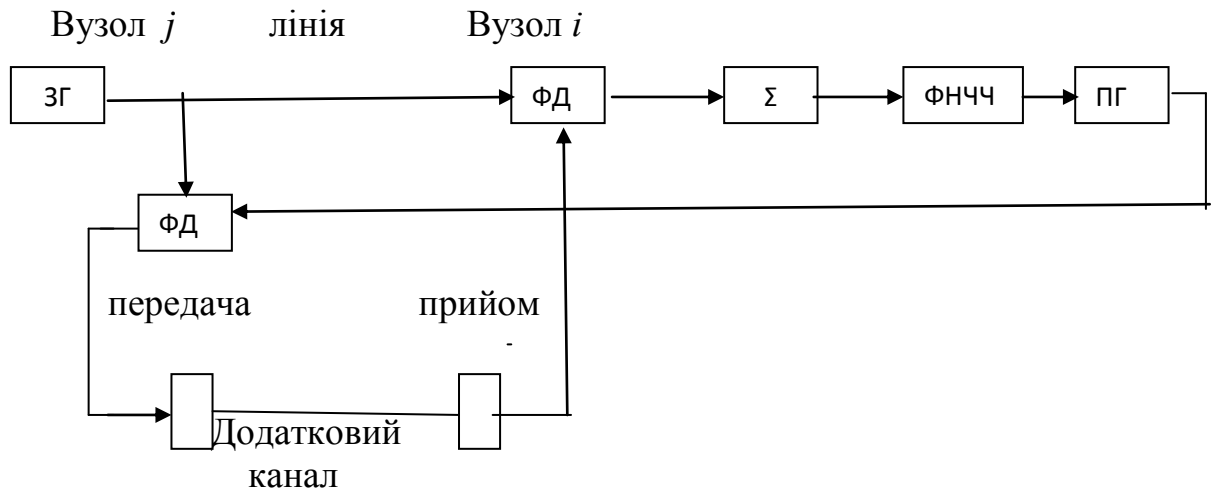
Рисунок 3.2 – Двокінцева синхронізація
