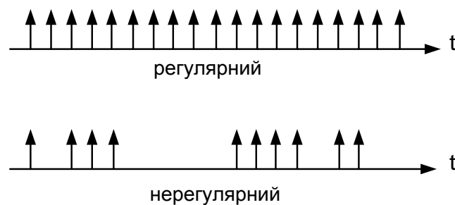
Рисунок 1.5 – Приклад регулярного та не регулярного синхросигналу
