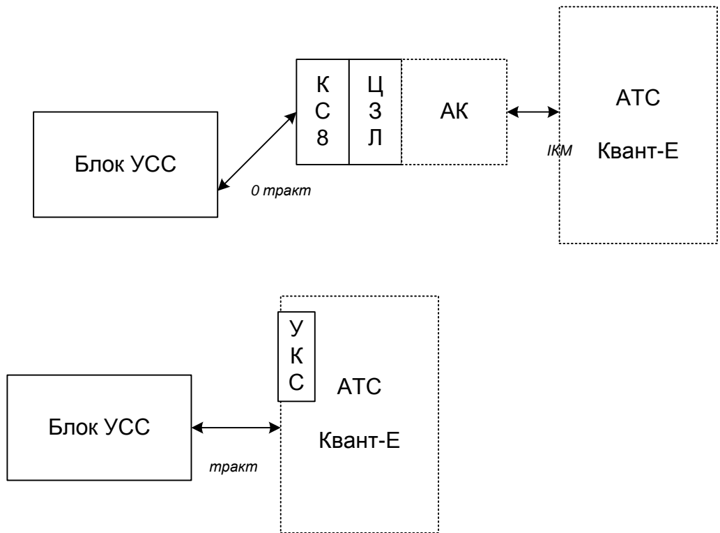
Рисунок 9.3 – Схема з'єднання блоку УСС з цифровою системою комутації «Квант-Е».
