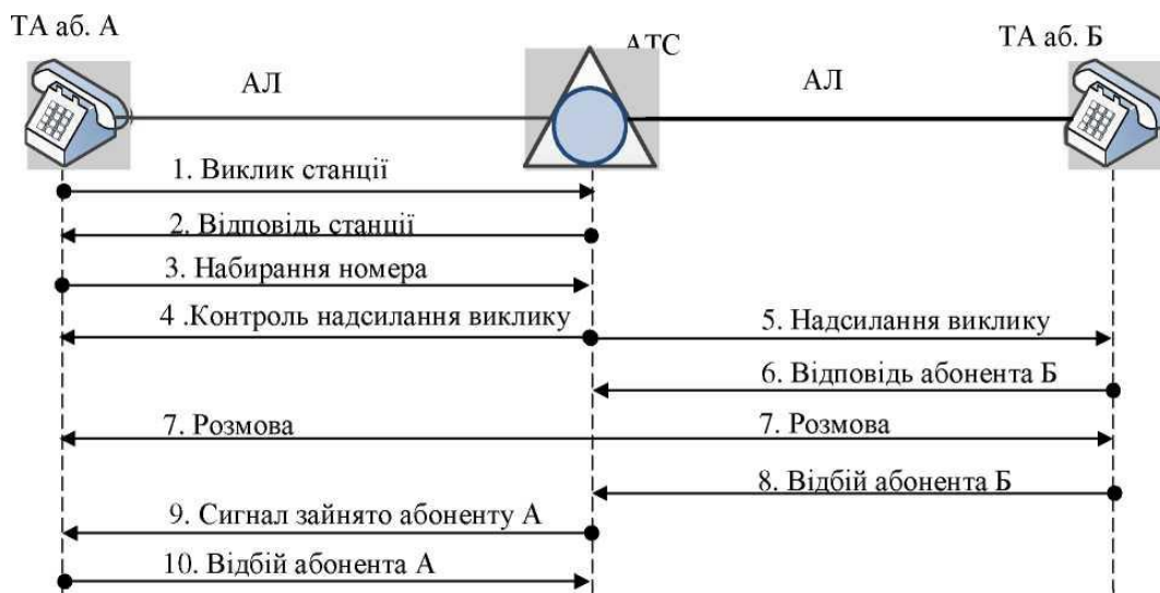
Рисунок 6.2 – Передавання сигналів на абонентській частині мережі
