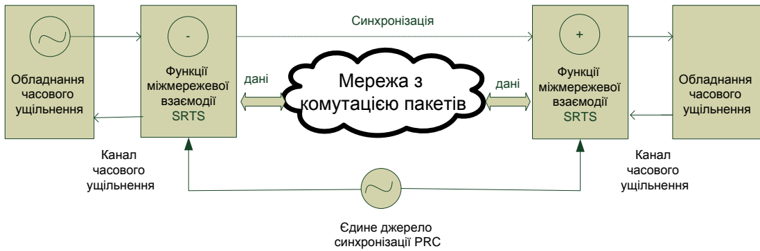
Рисунок 2.4 – Синхронізація з використанням власної тактової частоти абонентського обладнання
