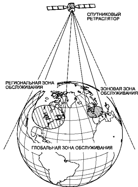
Рисунок 5.2 – Зони обслуговування ССЗ
