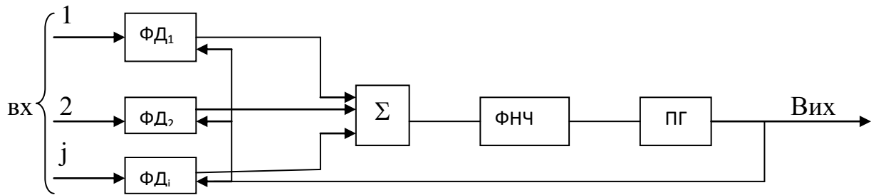
Рисунок 3.3 – Приклад однокінцевої взаємної синхронізації
