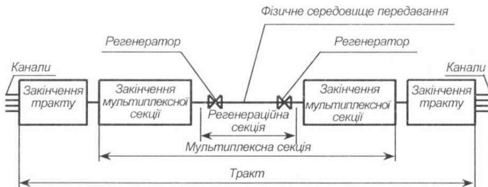
Рисунок 4.1 - Шари синхронної цифрової ієрархії
