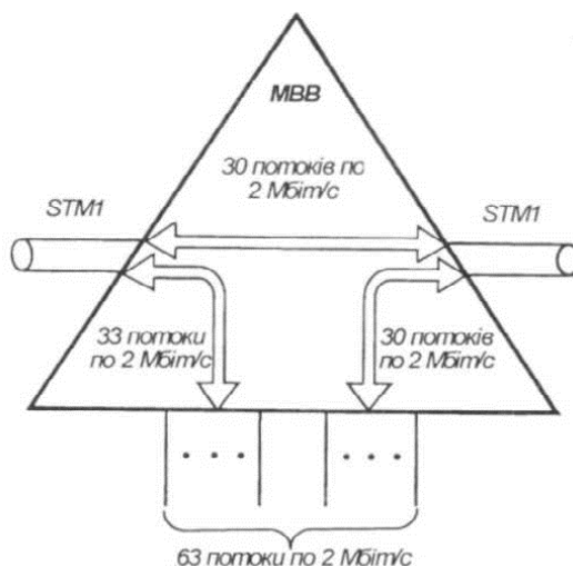
Рисунок 4.5 – Приклад схеми введення-виведення
