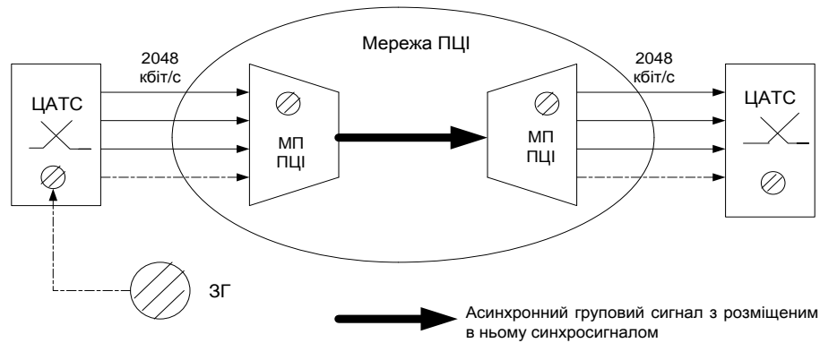
Рисунок 3.7 - Синхронізація двох цифрових вузлів комутації по лінії передавання ПЦІ (варіант 1).
