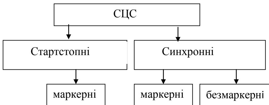
Рисунок 1.2 - Класифікація систем циклової синхронізації
