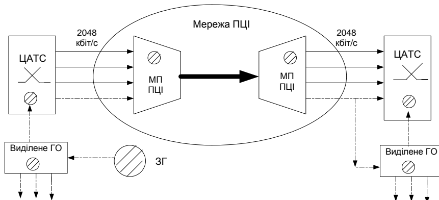
Рисунок 3.8 - Синхронізація двох цифрових вузлів комутації по лінії передавання ПЦІ (варіант 2).
