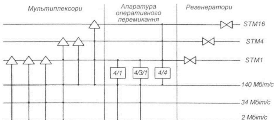
Рисунок 4.9 - Основні види апаратури синхронної цифрової ієрархії
