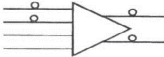
Рисунок 4.7 – Конфігурація, що забезпечує поєднання функцій концентратора та мультиплексора введення-виведення
