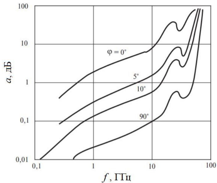
Рис. 3.2. Частотні залежності сумарного молекулярного послаблення радіосигналу
