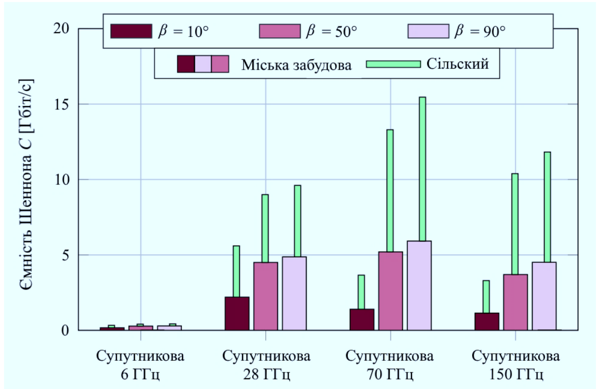
Рис. 3.6. Ємність Шеннона для ліній зв'язку супутникових конфігурацій різних частот для різних кутів елевації супутників \beta . S/N = 0 дБ, G_{\text{ГХ}} = 50 дБ, h = 300 км (LEO). Сценарій щільної міської забудови/сільської місцевості для широкого/вузького променю
