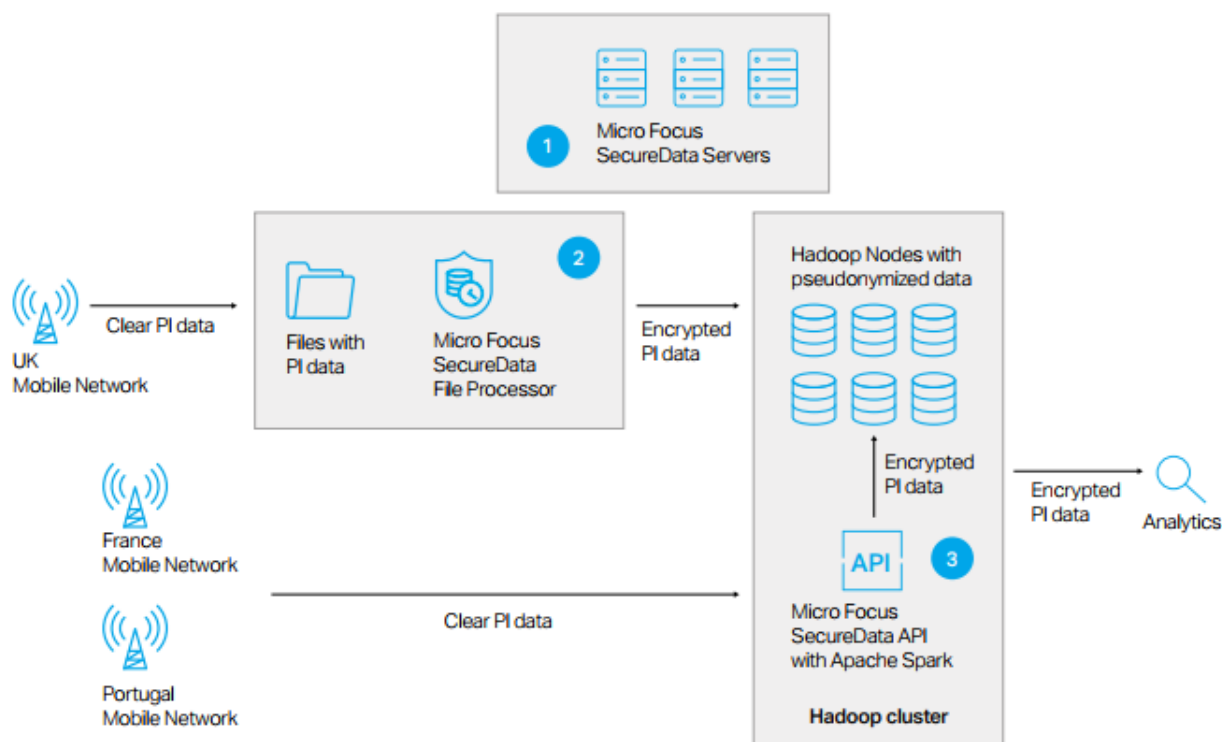
Рис 3.1. Архітектура де-ідентифікації даних у Hadoop
