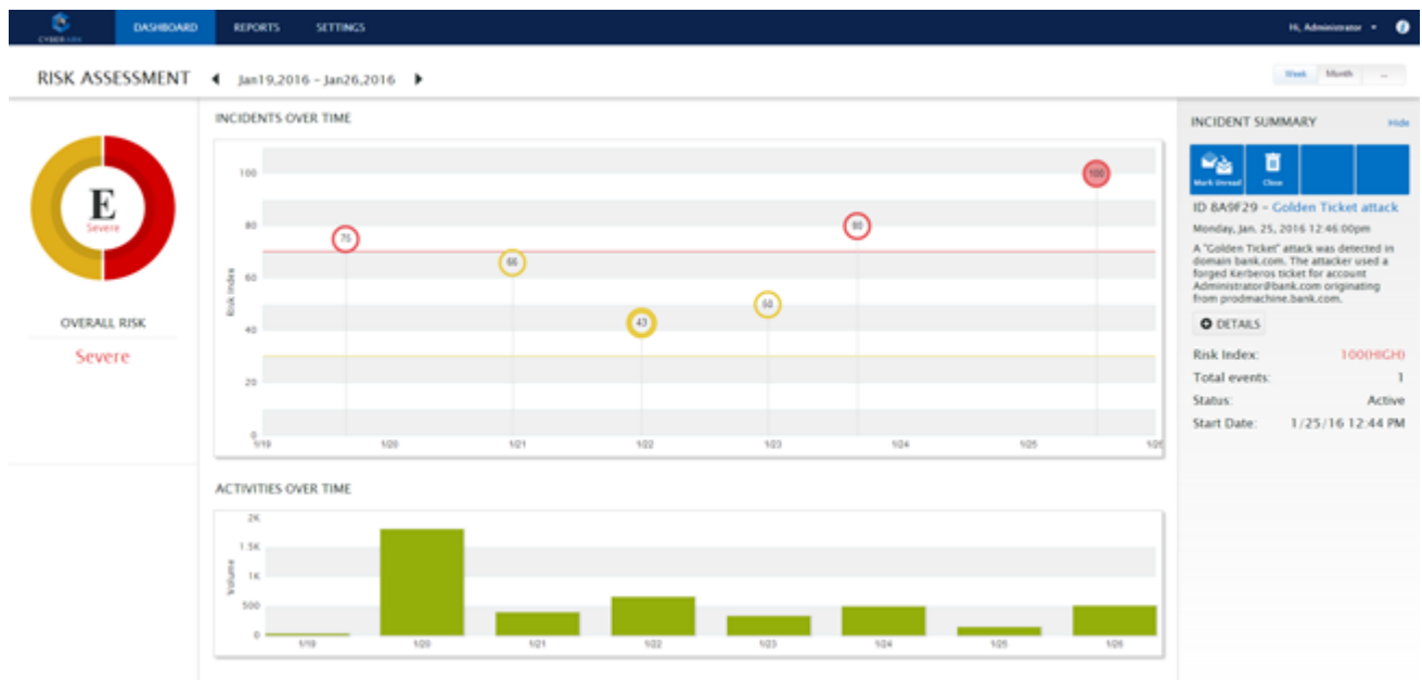
Рис 3.4. Веб-консоль CyberArk Privileged Threat Analytics
