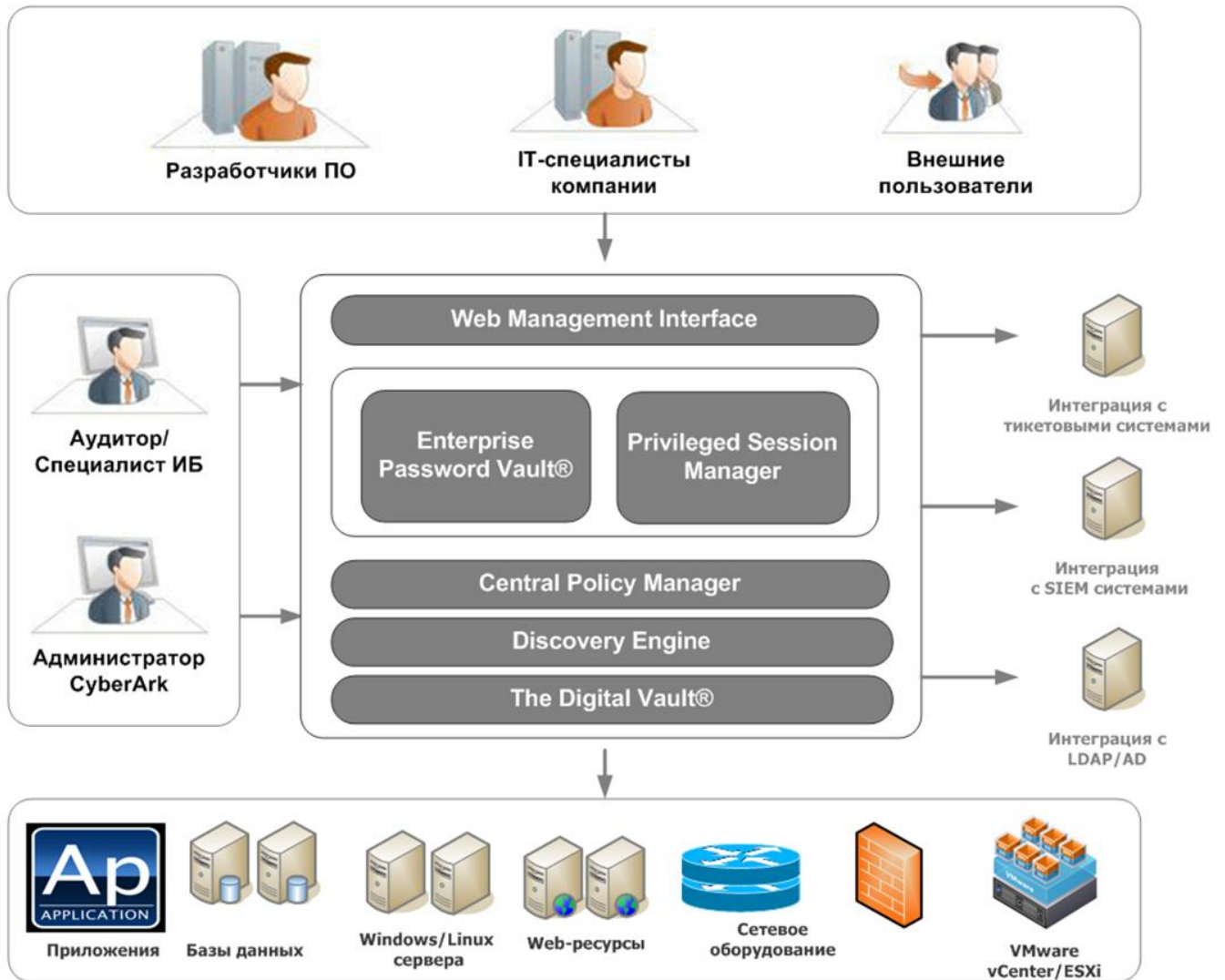
Рис.2.10. Архітектура рішення
