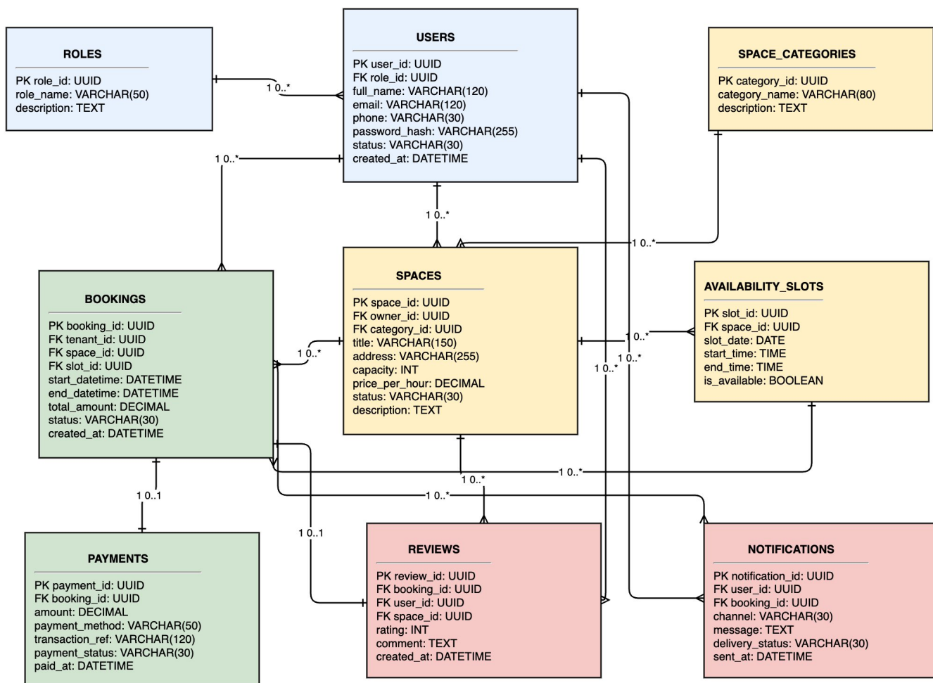
Рис.2.4.Логічна модель бази даних веб-платформи бронювання оренди приміщень
