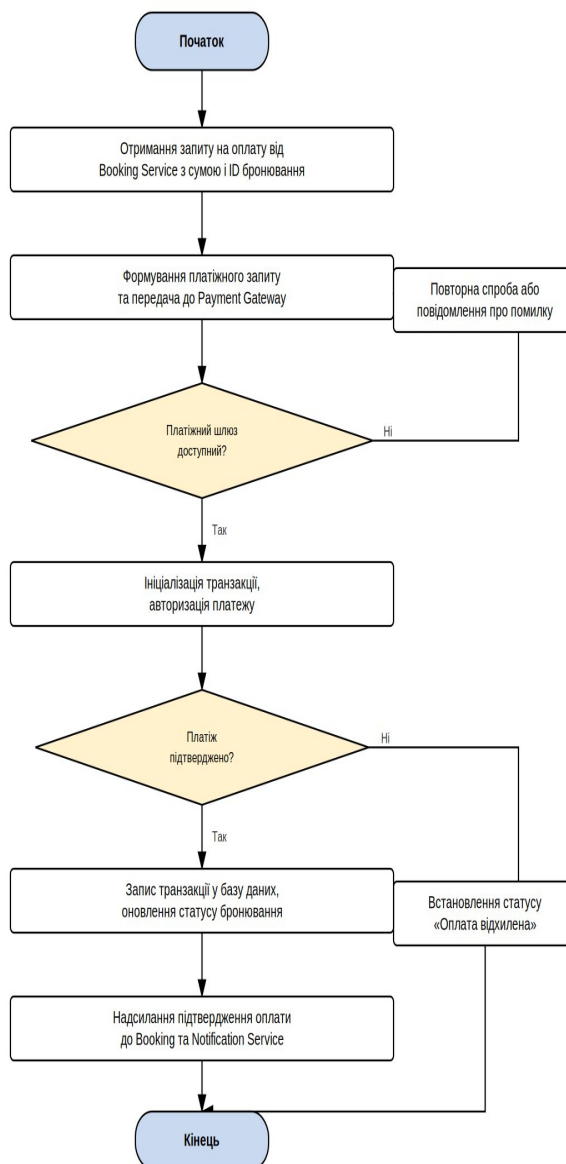
Рис.3.5.Блок-схема алгоритму оброблення платежу
