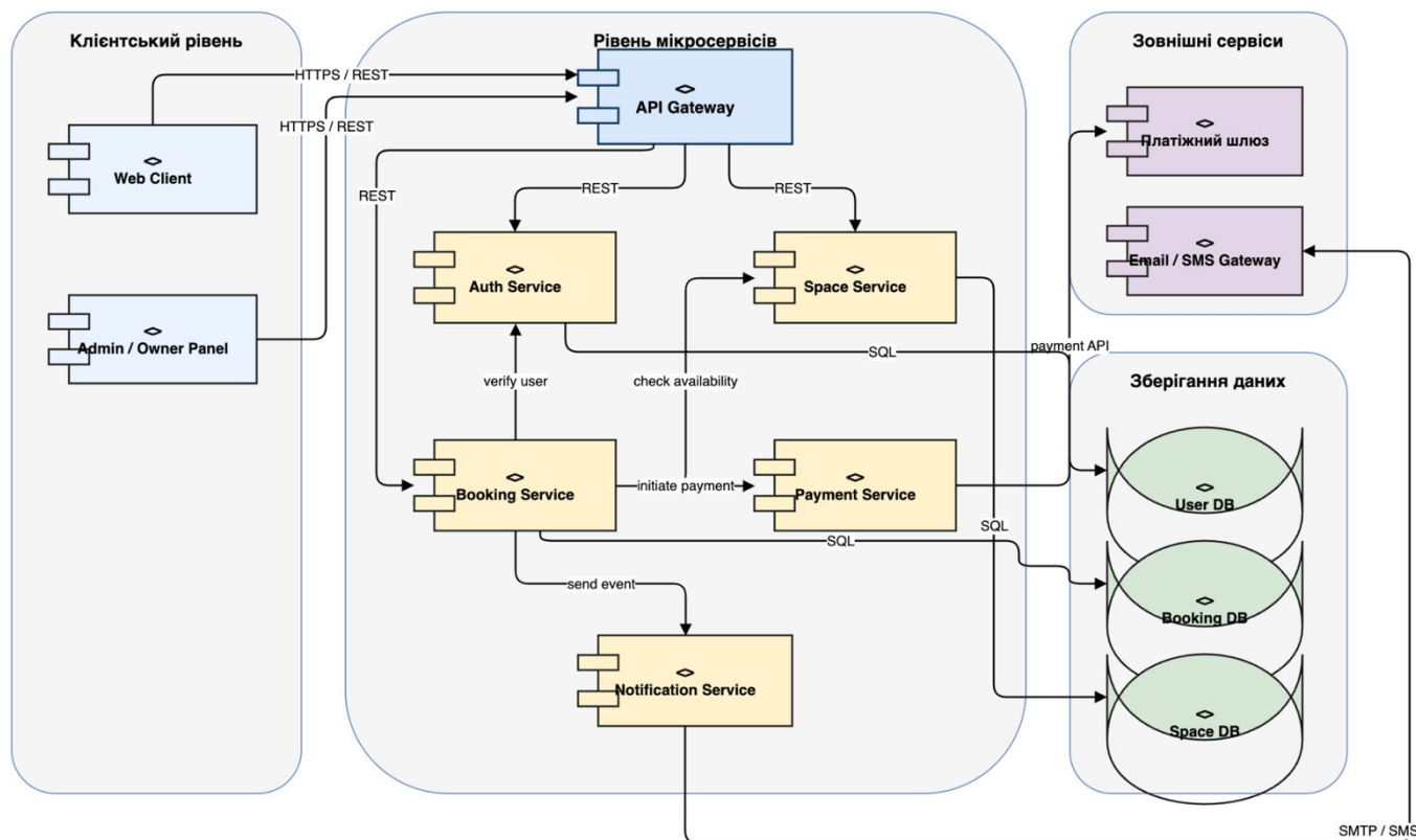
Рис.3.1.Структурна схема реалізації веб-платформи бронювання оренди приміщень
