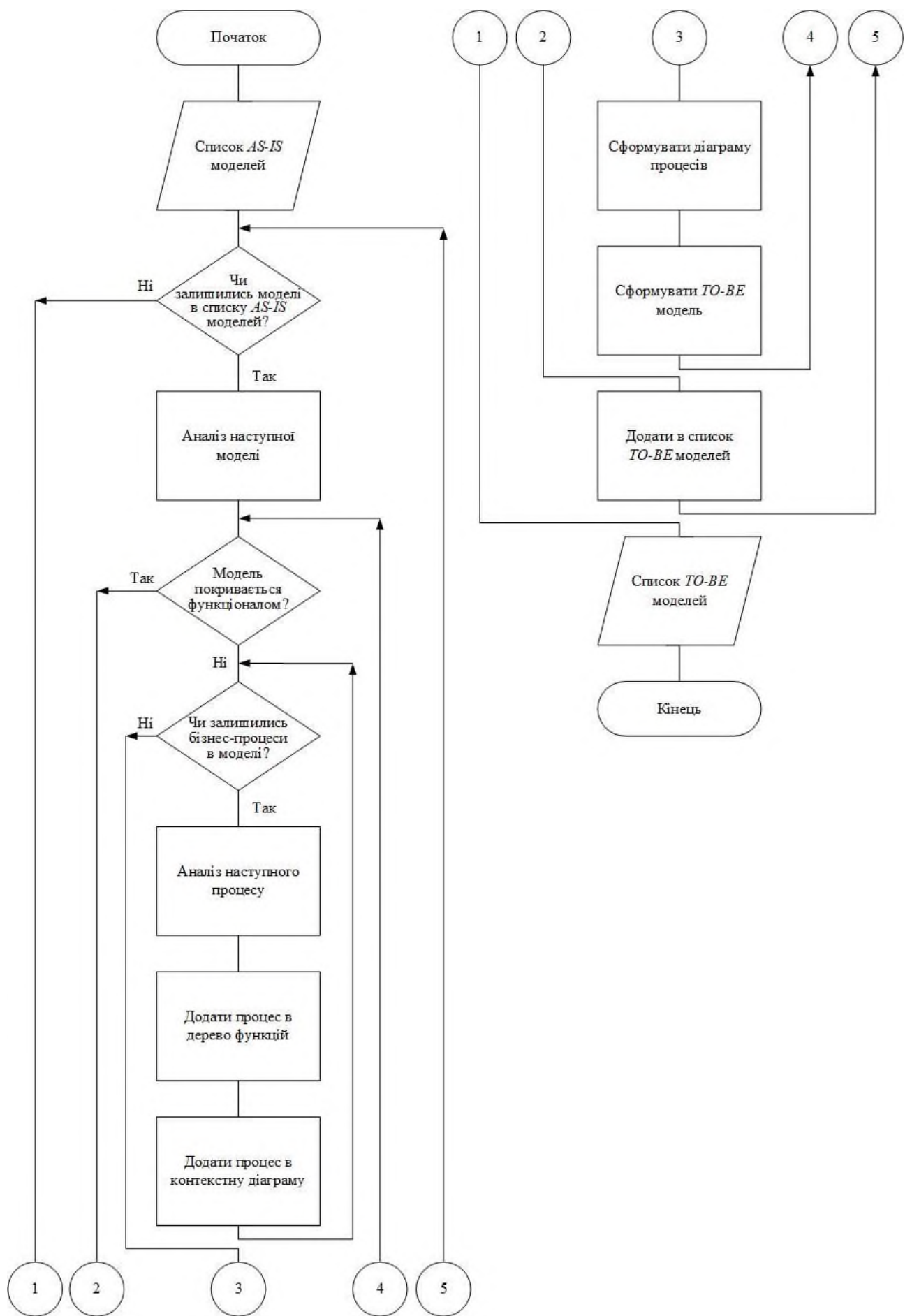
Рис. 3.5. Схема алгоритму формування TO-BE моделей
