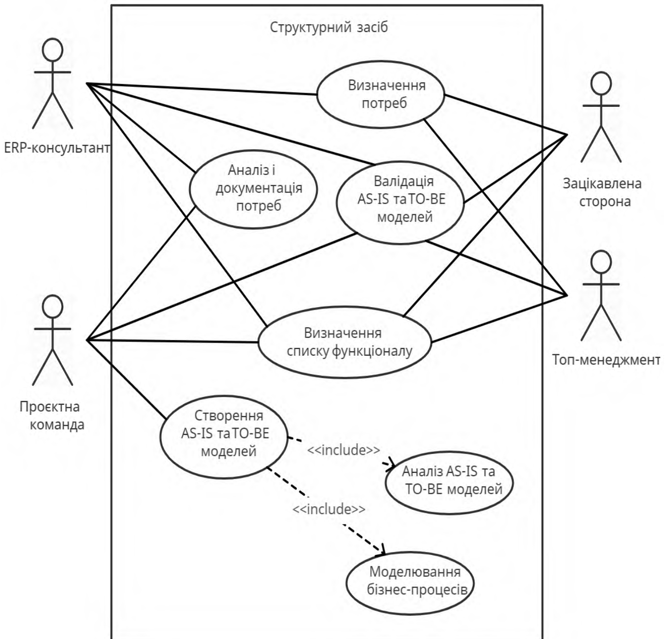
Рис. 3.3. Діаграма прецедентів
